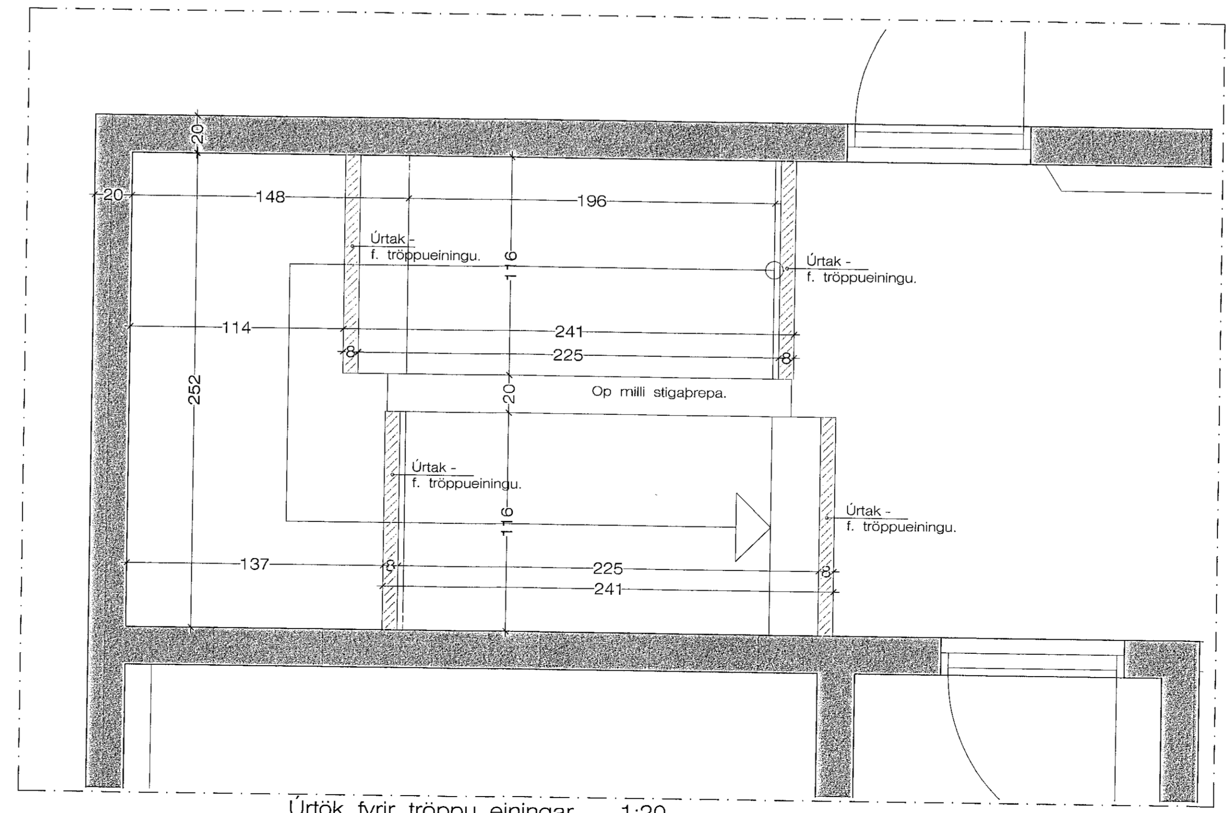
Úrtök fyrir tröppu einingar. 1:20
