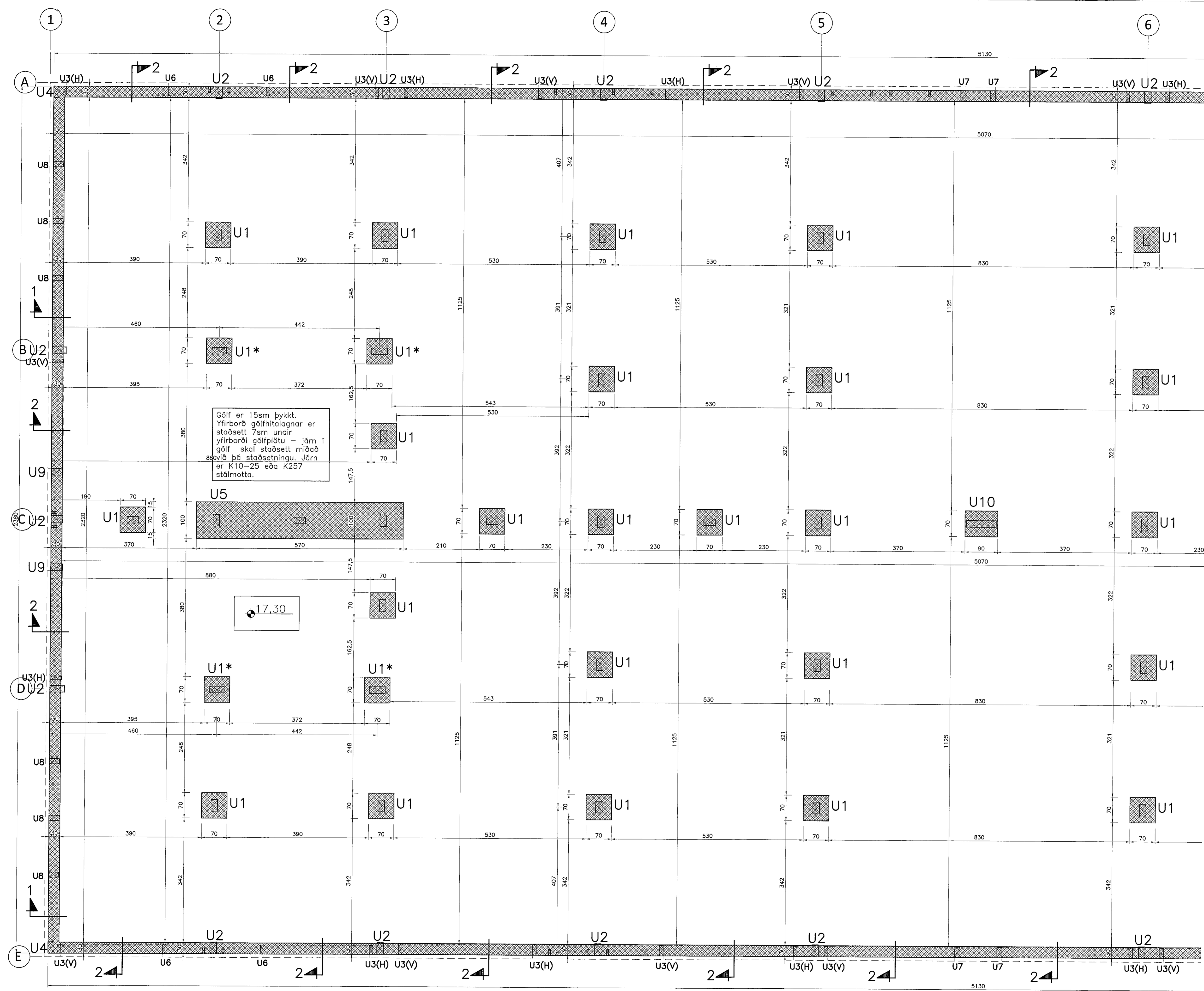
Grunnmynd undirstaða (milli lína 1-6) 1:50
