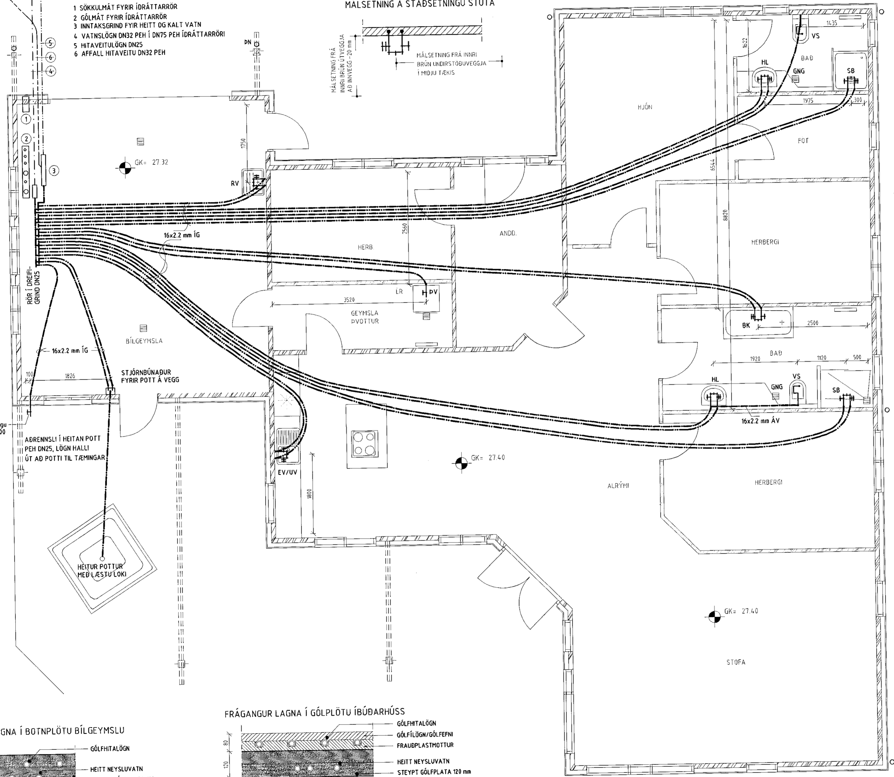
VATNSLAGNIR GRUNNMYND 1:50
