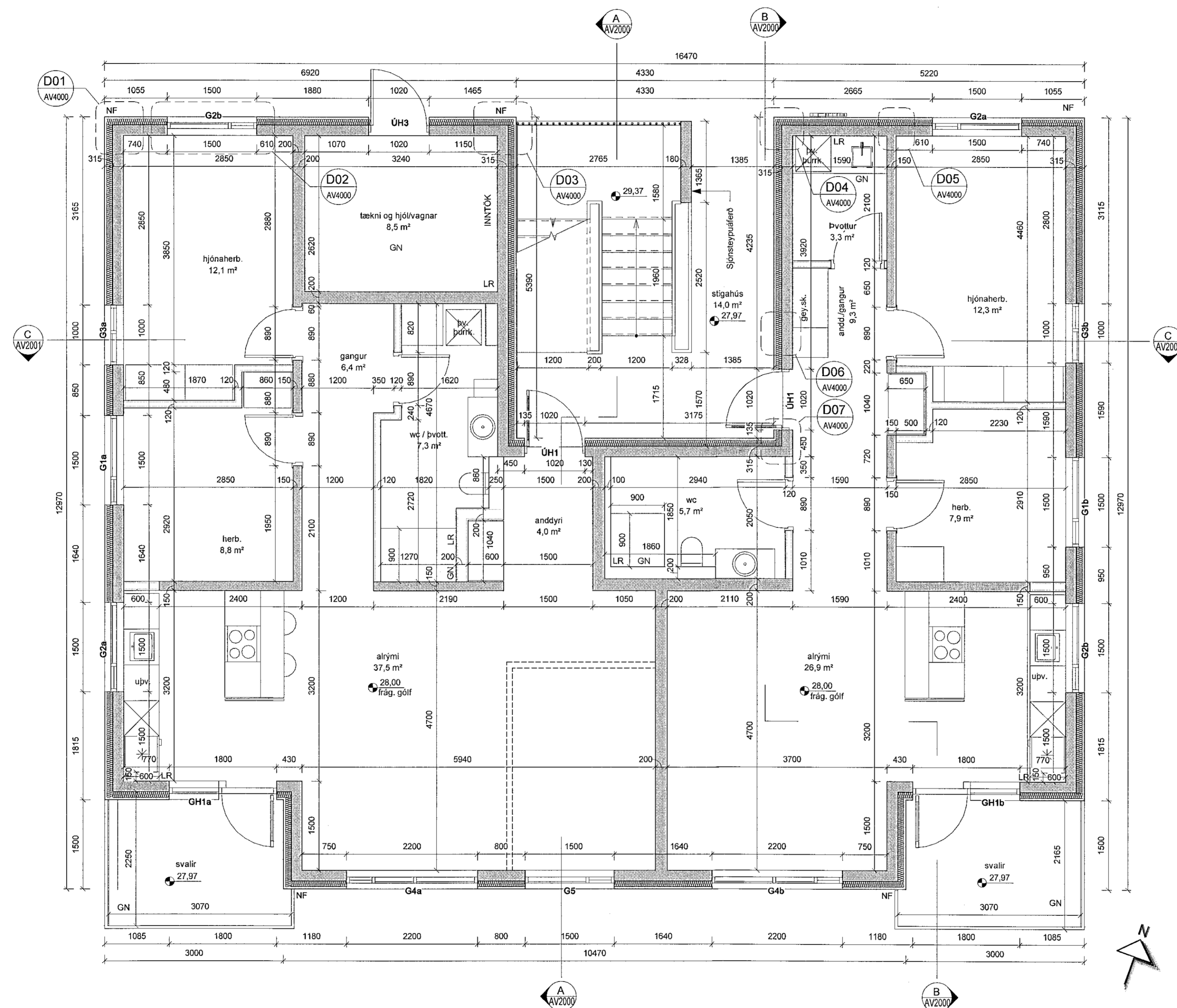
2.HÆÐ mkv: 1 : 50
