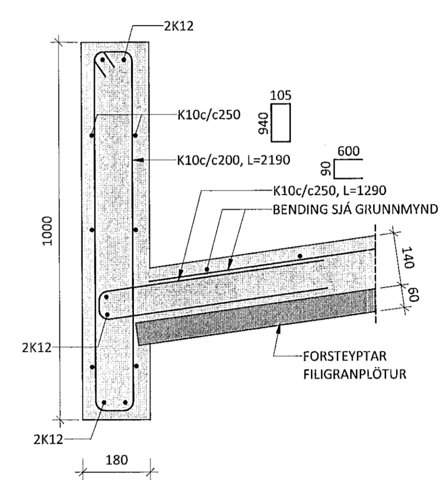
P8 M 1 : 10
