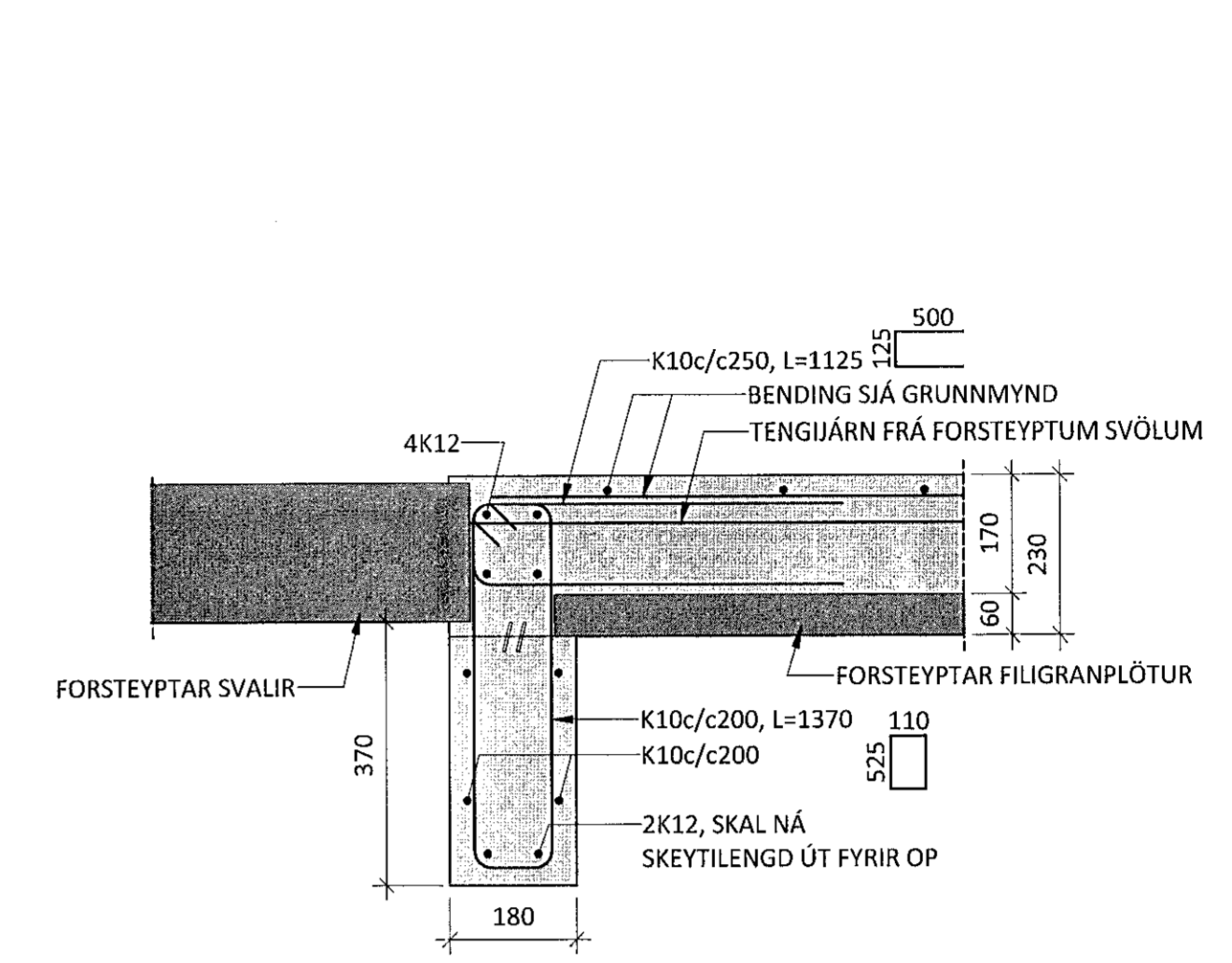
P4 M 1 : 10
