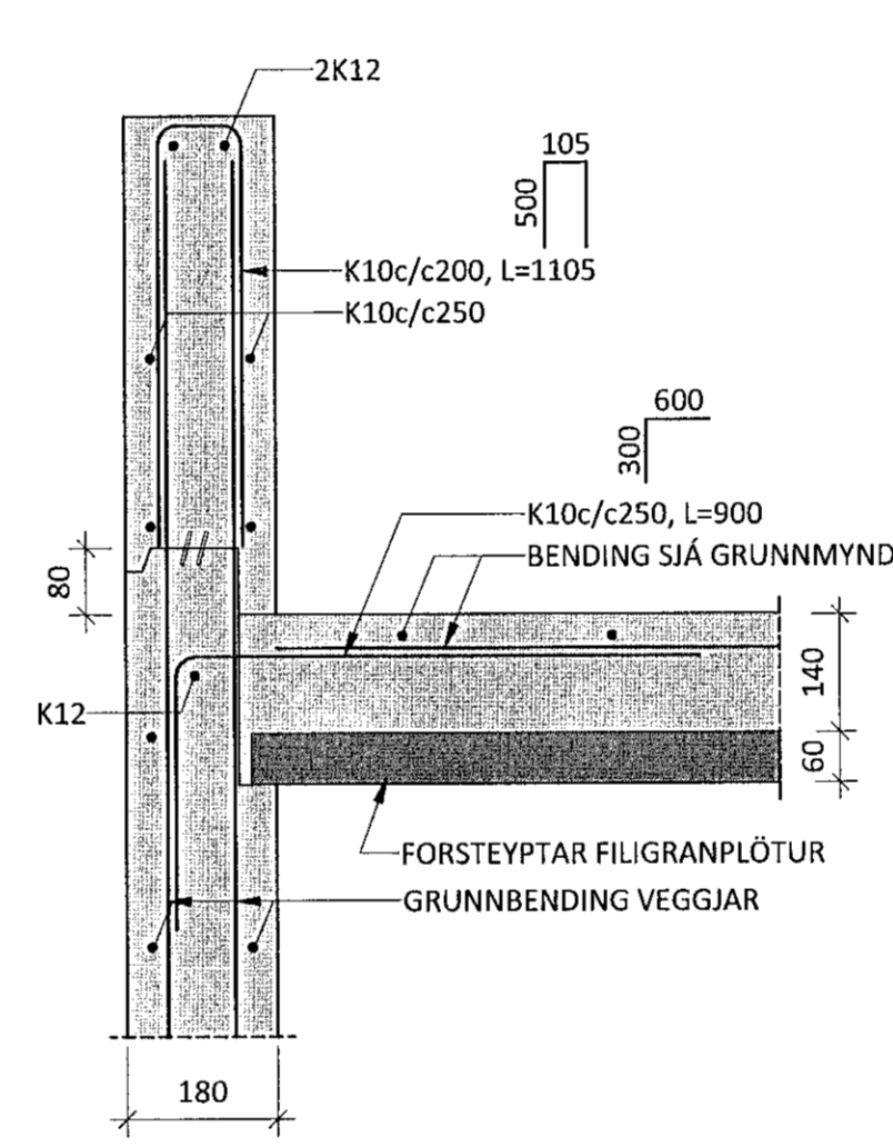
P7 M 1 : 10
