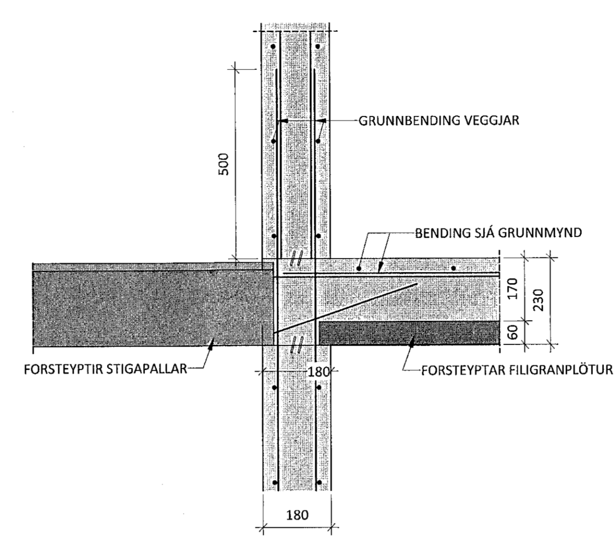
P3 M 1 : 10
