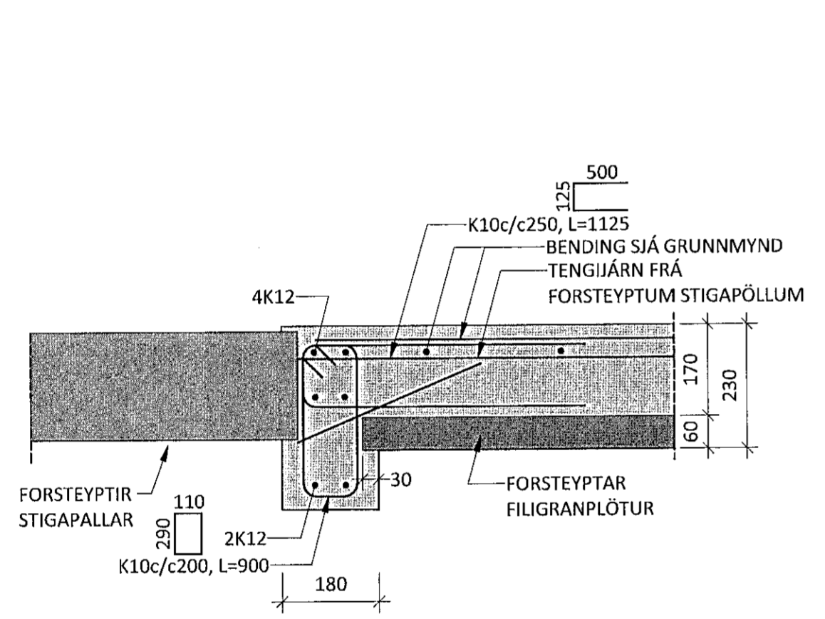
P5 M 1 : 10
