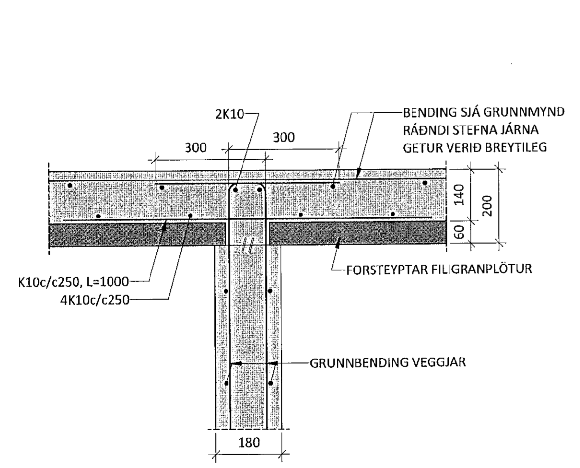
P9 M 1 : 10
