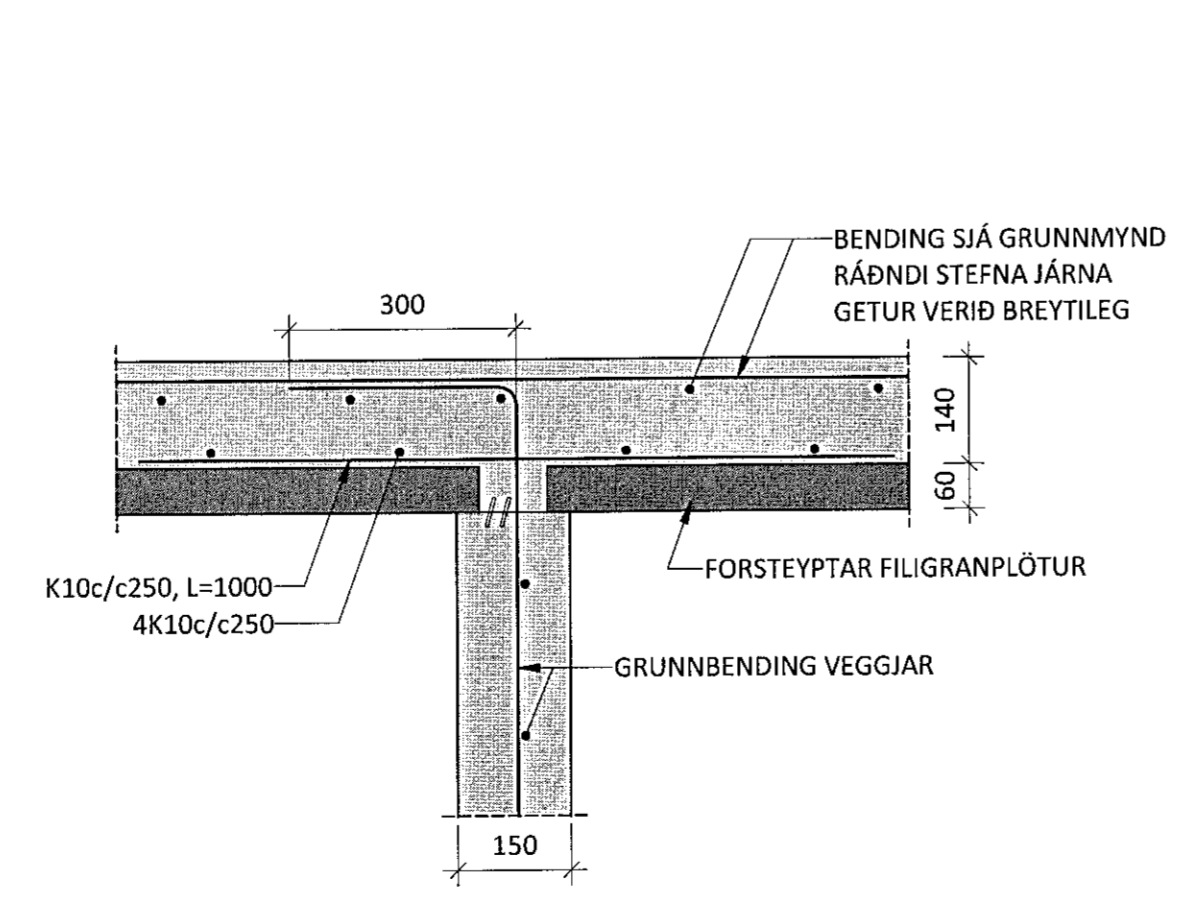
P10 M 1 : 10
