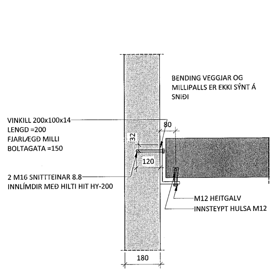
P2 M 1 : 10
