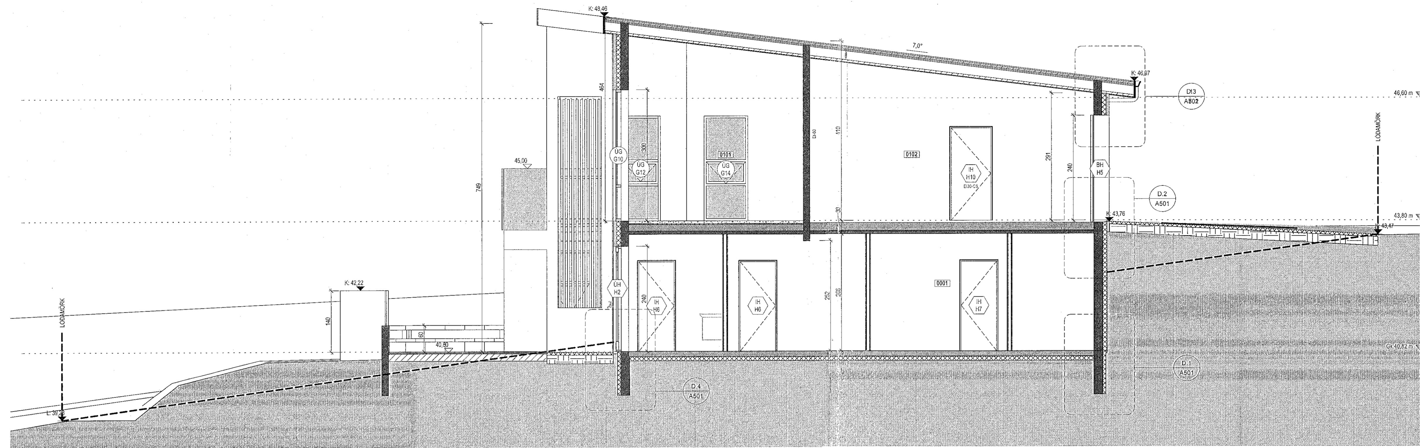
Snið 1 1:50
