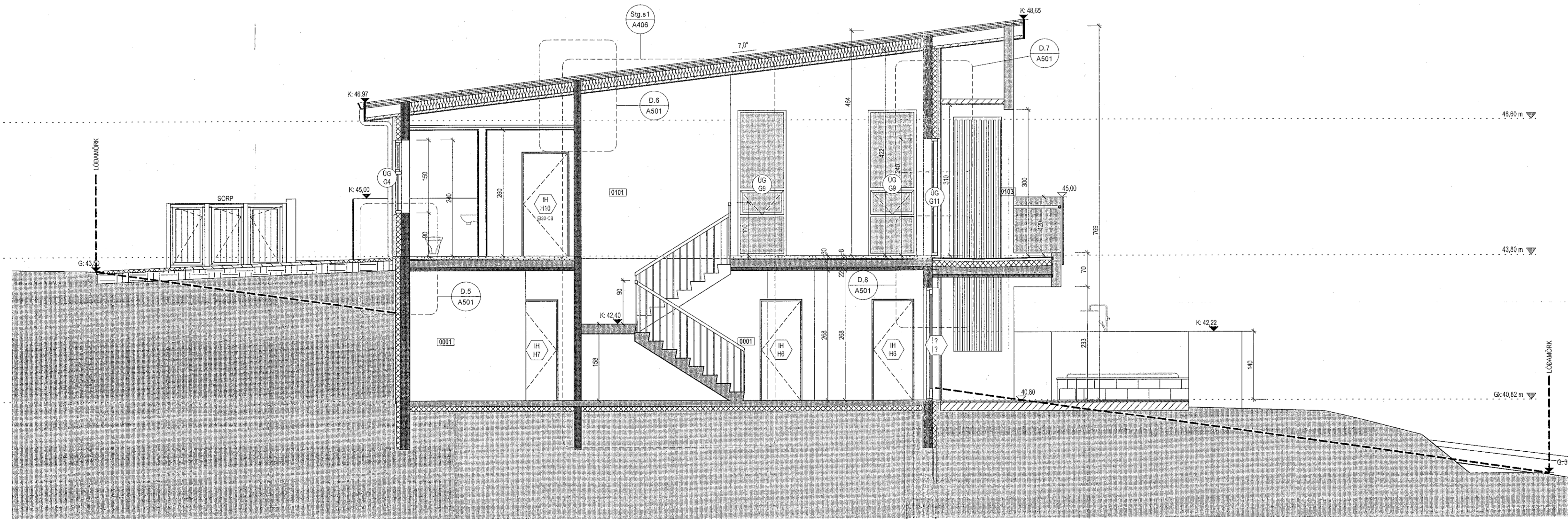
Snið 2 1:50
