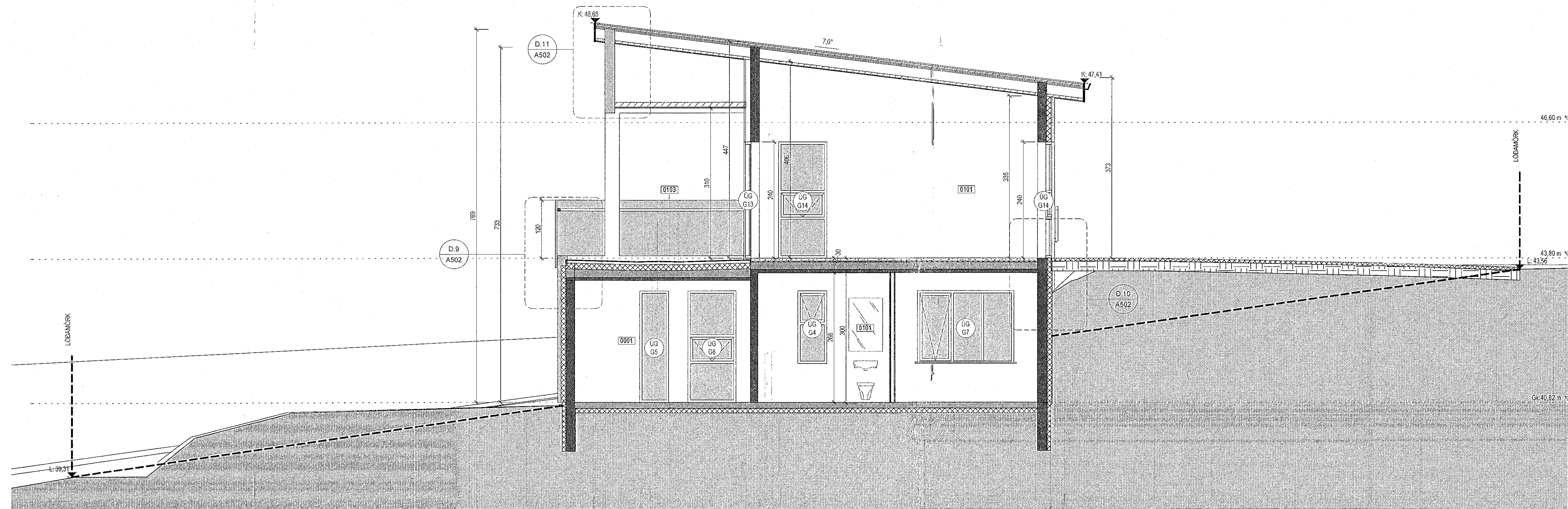
Snið 3 1:50
