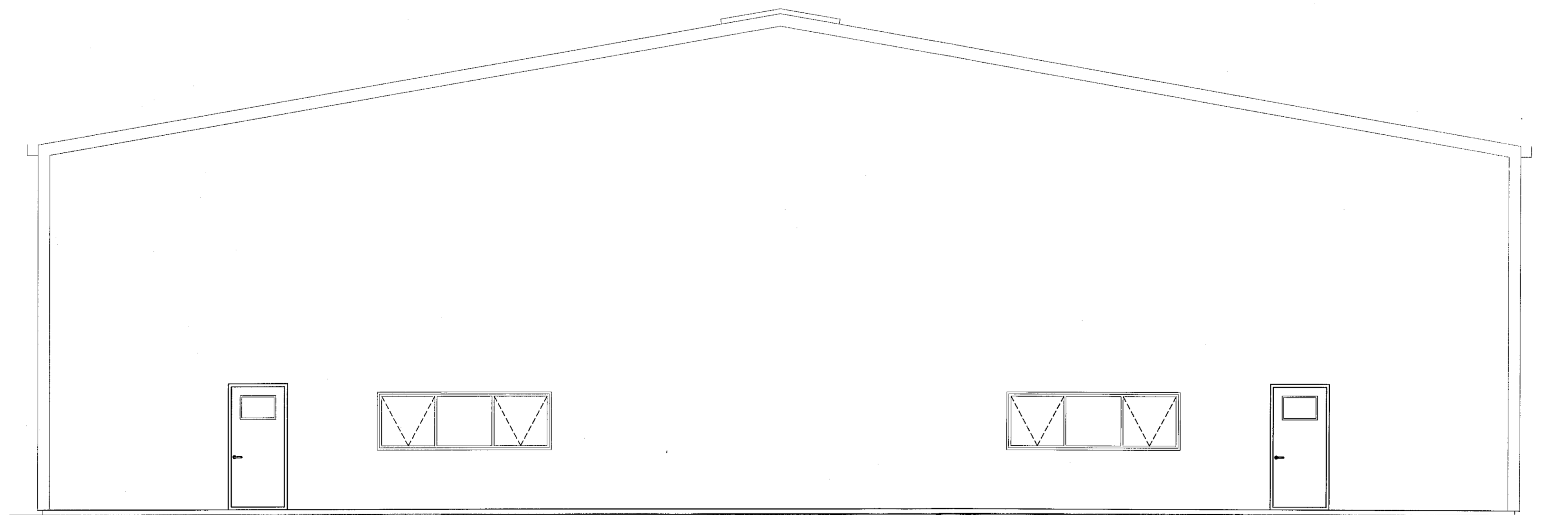
Norð vestur gafi 1:50
