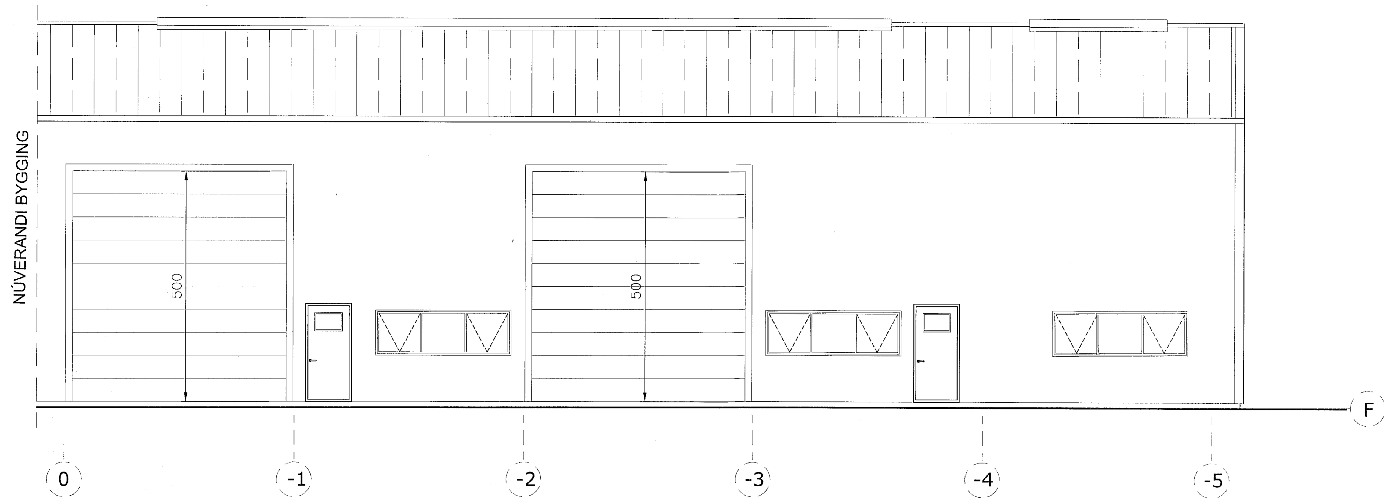
Norð vestur hlið 1:50.
