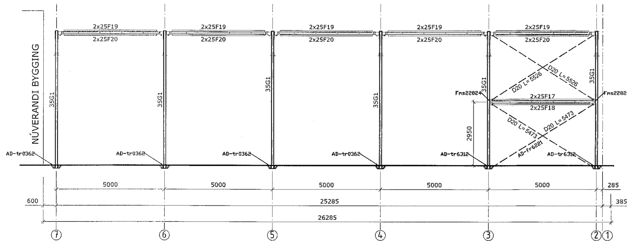
langveggur í línu A (Stálburðarvirki)
