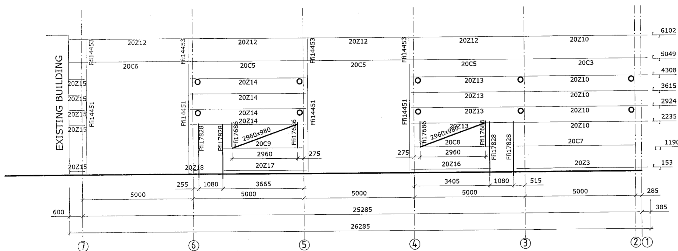
Langveggur í línu A (vegglangbönd)
