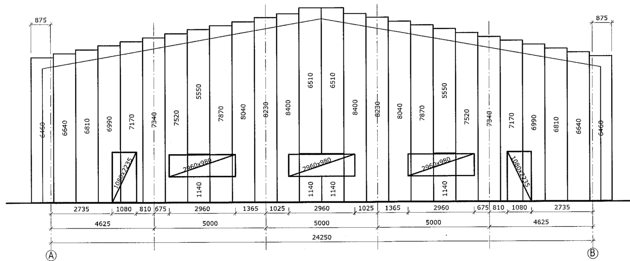
Gafelveggur í línu 1 (Klæðning, steinullar samlokur)
