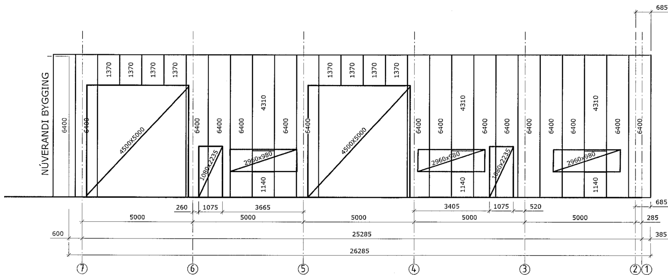
Langveggur í línu A (Klæðning, steinullar samlokur)
