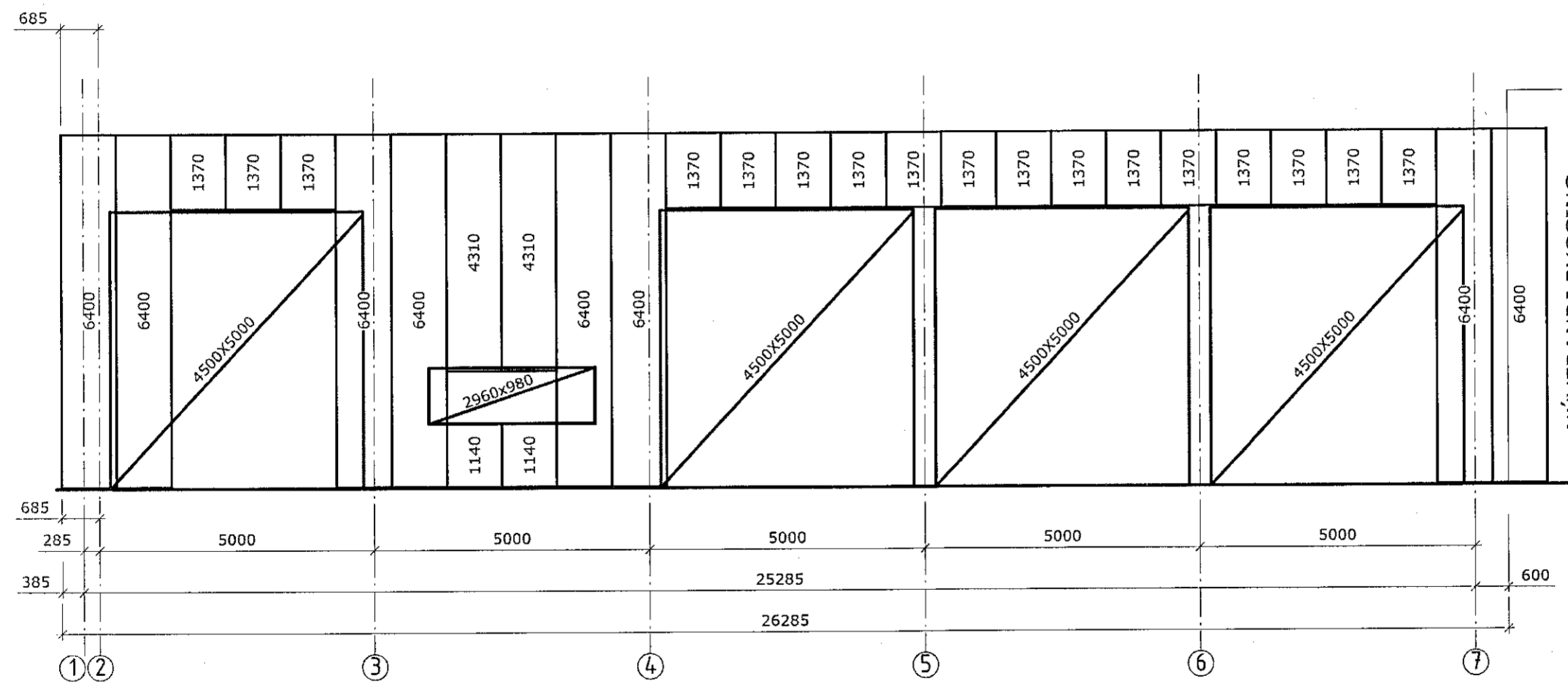
Langveggur í línu B (Klæðning, steinullar samlokur)
