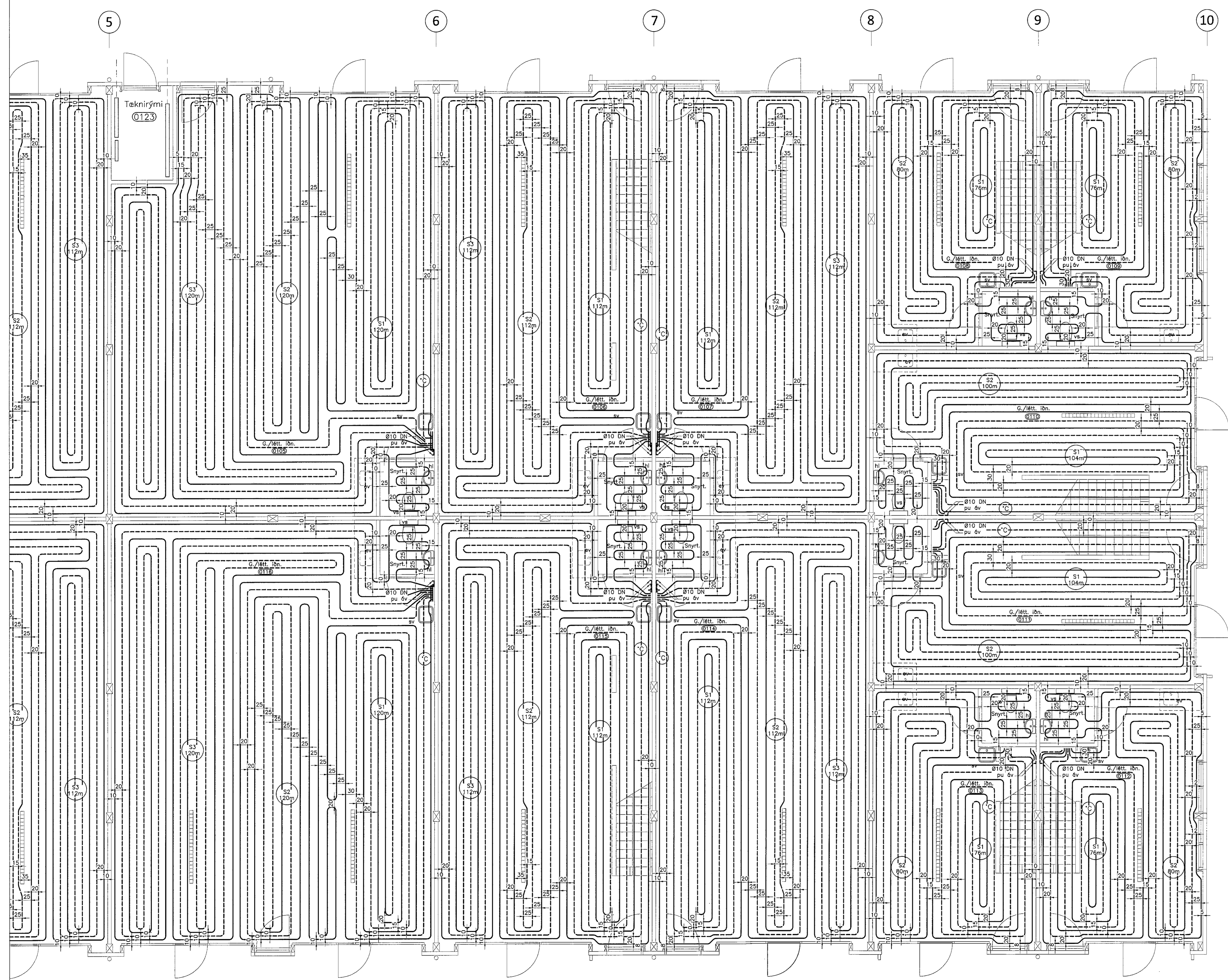
Gölfhitalagnir 1. hæðar (5-10) 1:50
