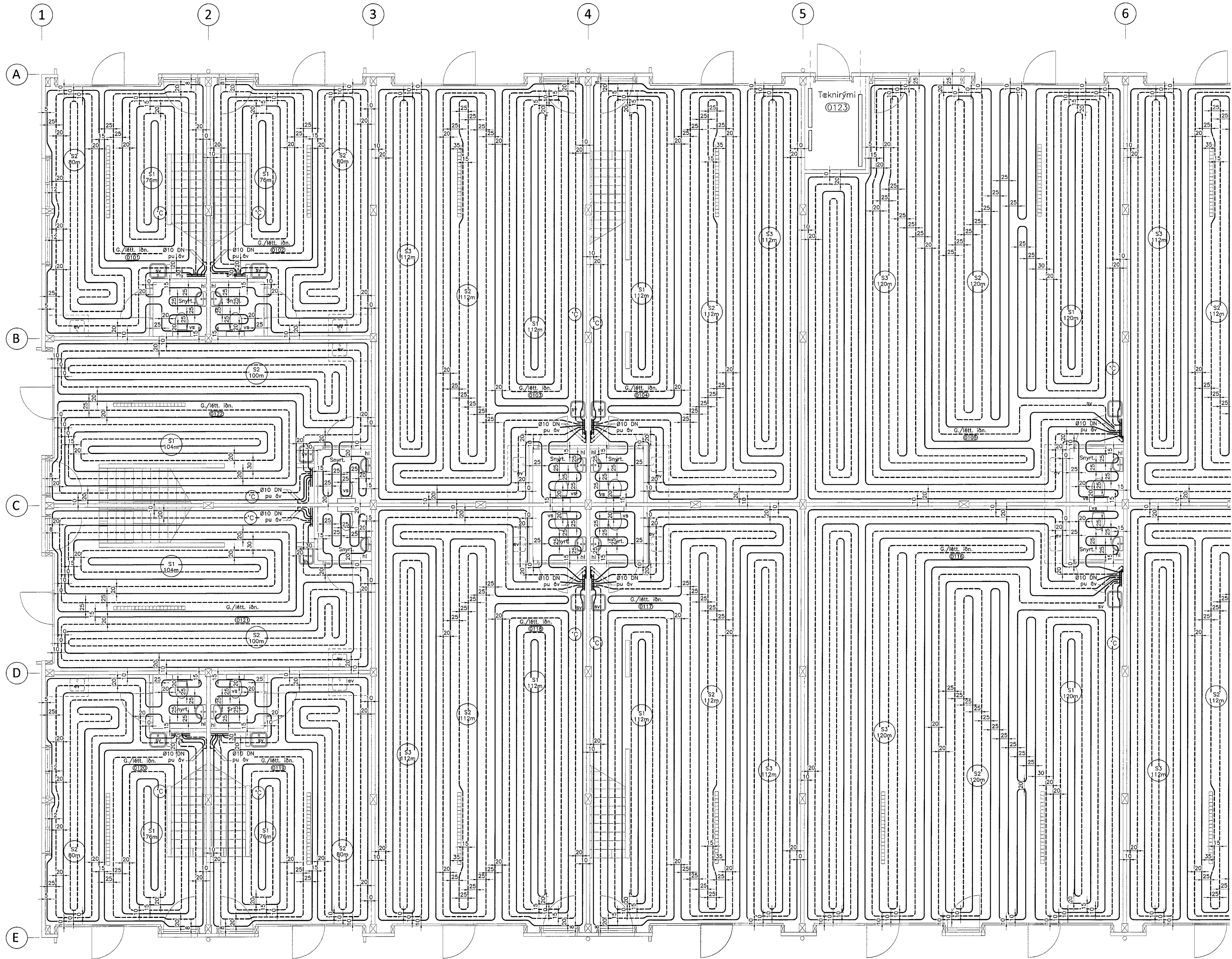
Gölfhitalagnir 1. hæðar (1-6) 1:50
