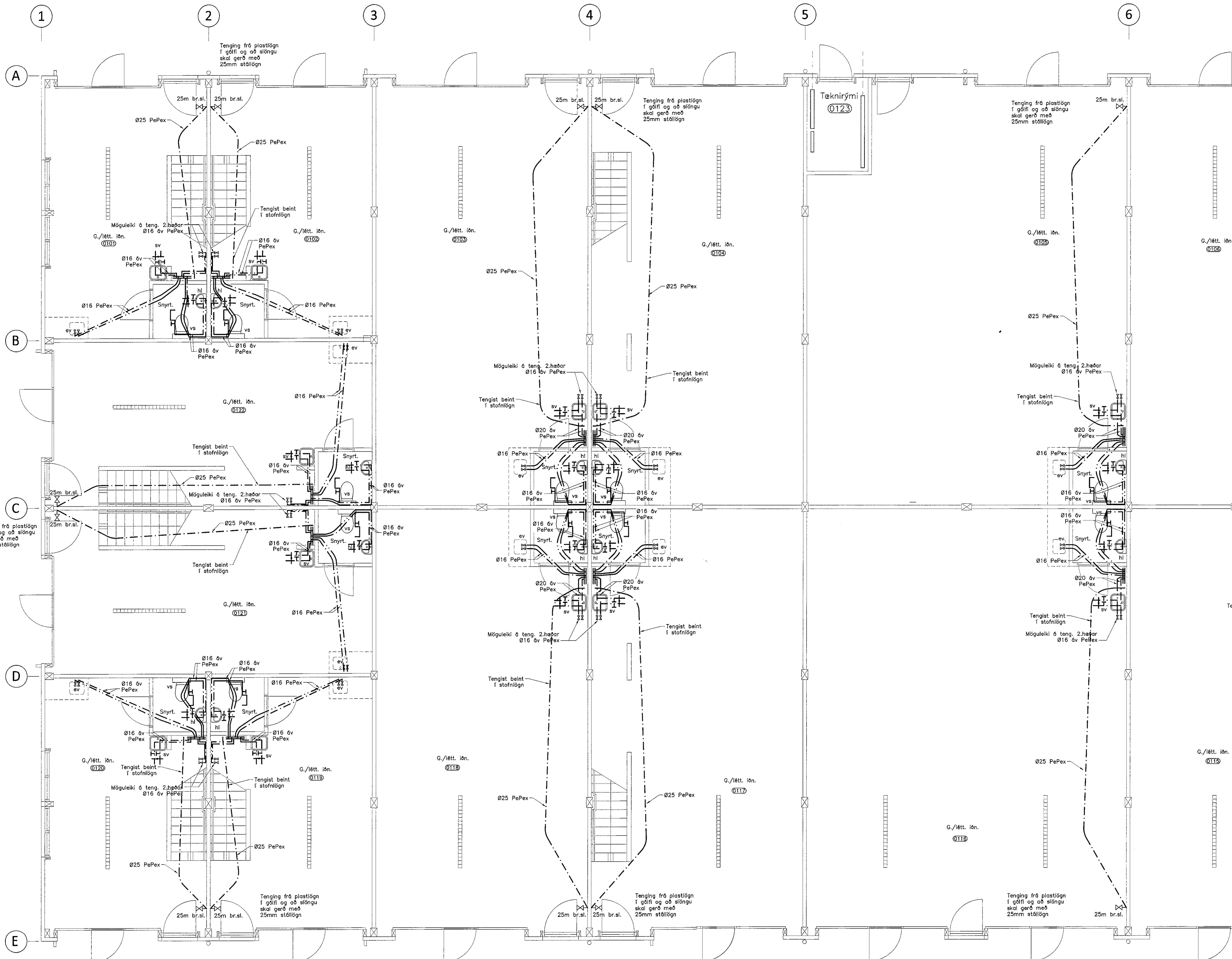
Neysluvatnslagnir 1. hæðar (1-6) 1:50
