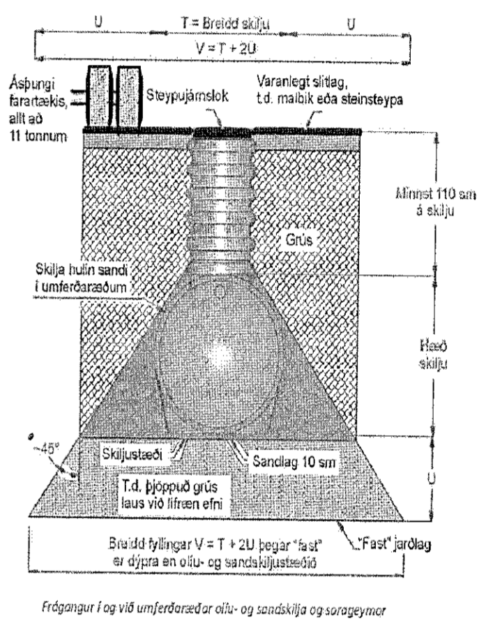
Sníð í brunn og lagdir. 1:20.
