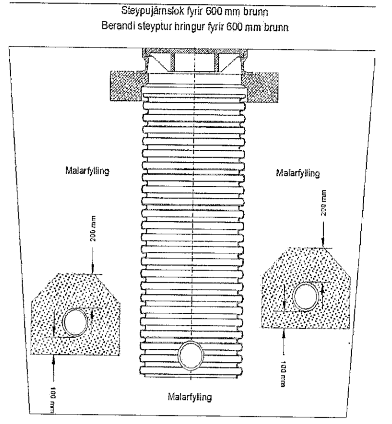
Sníð í brunn og lagdir. 1:20.
