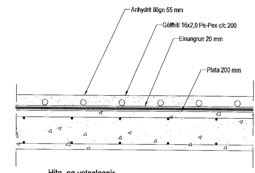
Hita- og vatnslagnir, Snið í milliþlotu, 1:10
