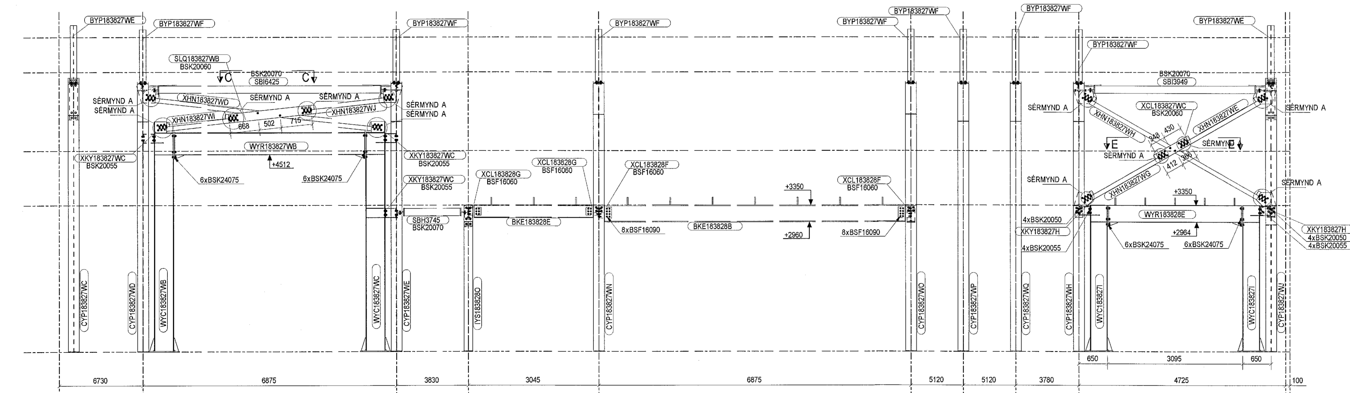
ÁS 5 - (UTANDYRA) MÆLIKV.: M 1:50
