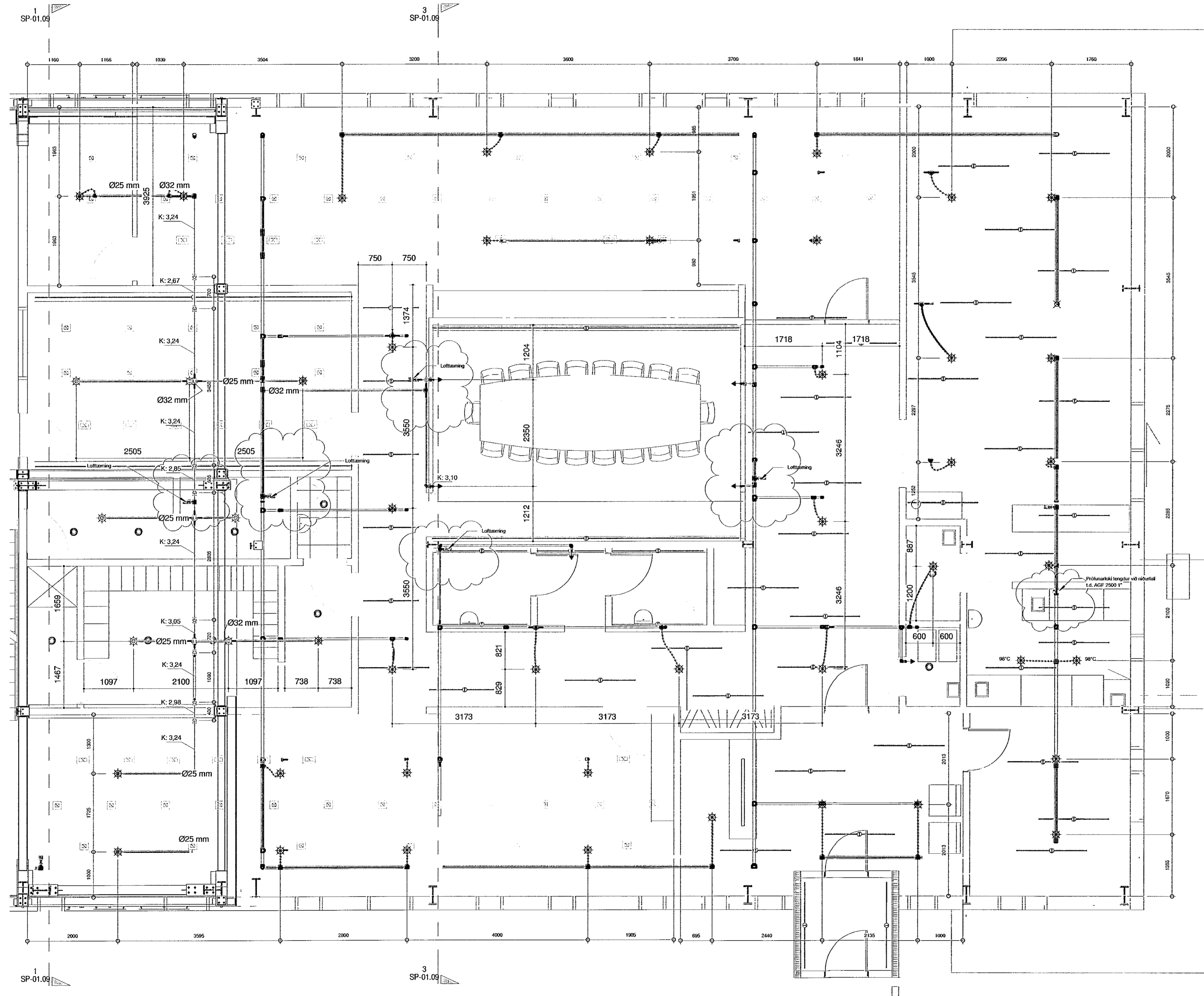
1. hæð kerfi í niðurteknum loftum skrifstofur mkv: 1 : 50
