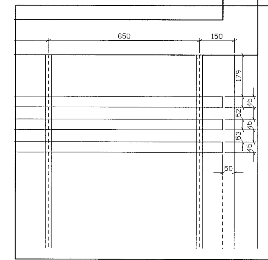
Deili C mál 1:10
