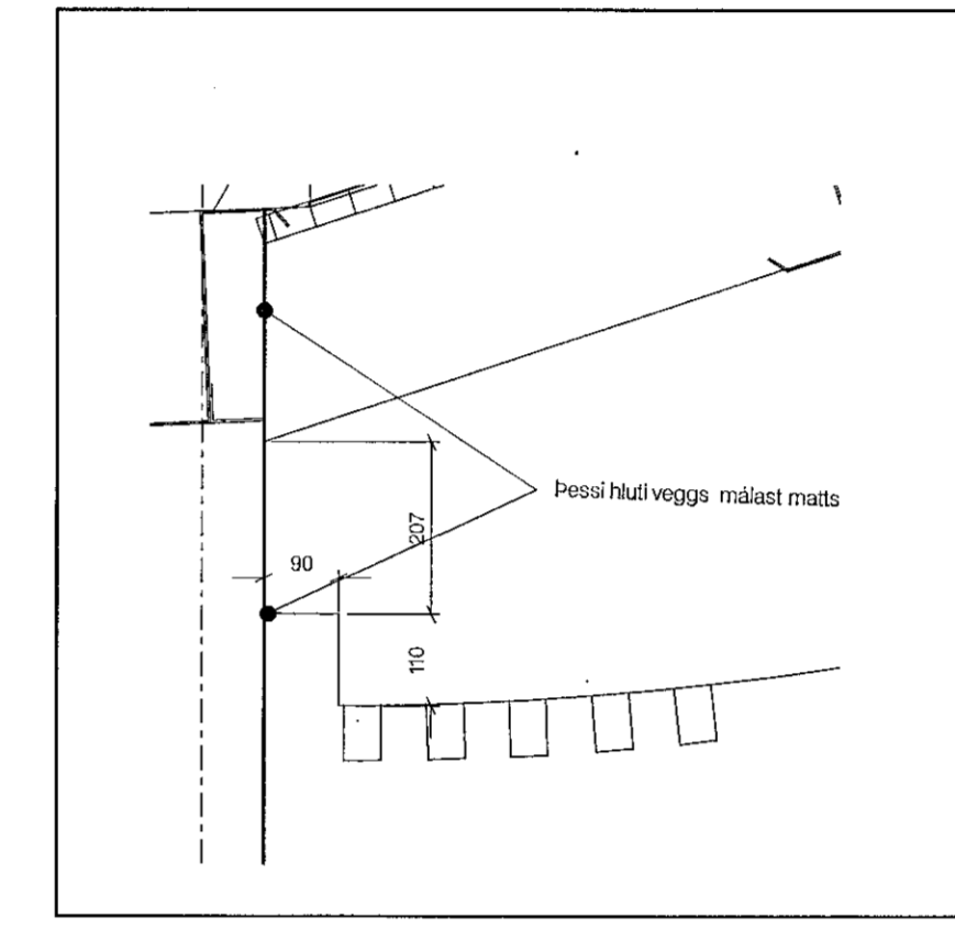
Deili B mál 1:10
