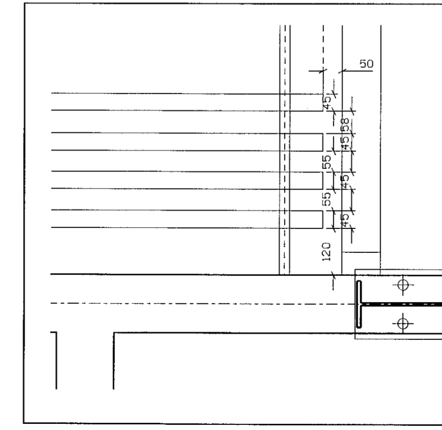
Deili D mál 1:10
