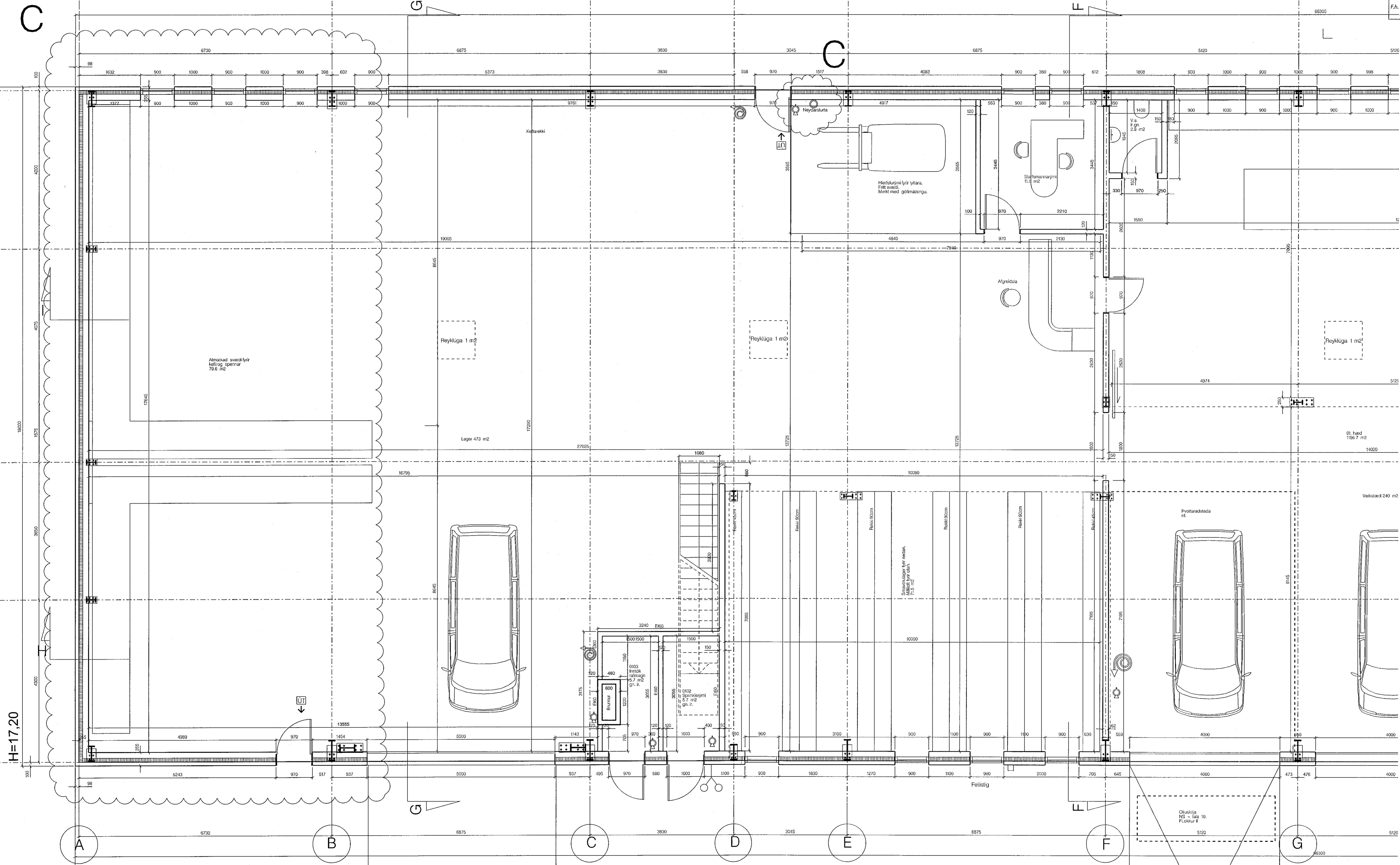
Grunnmynd 1. hæð
