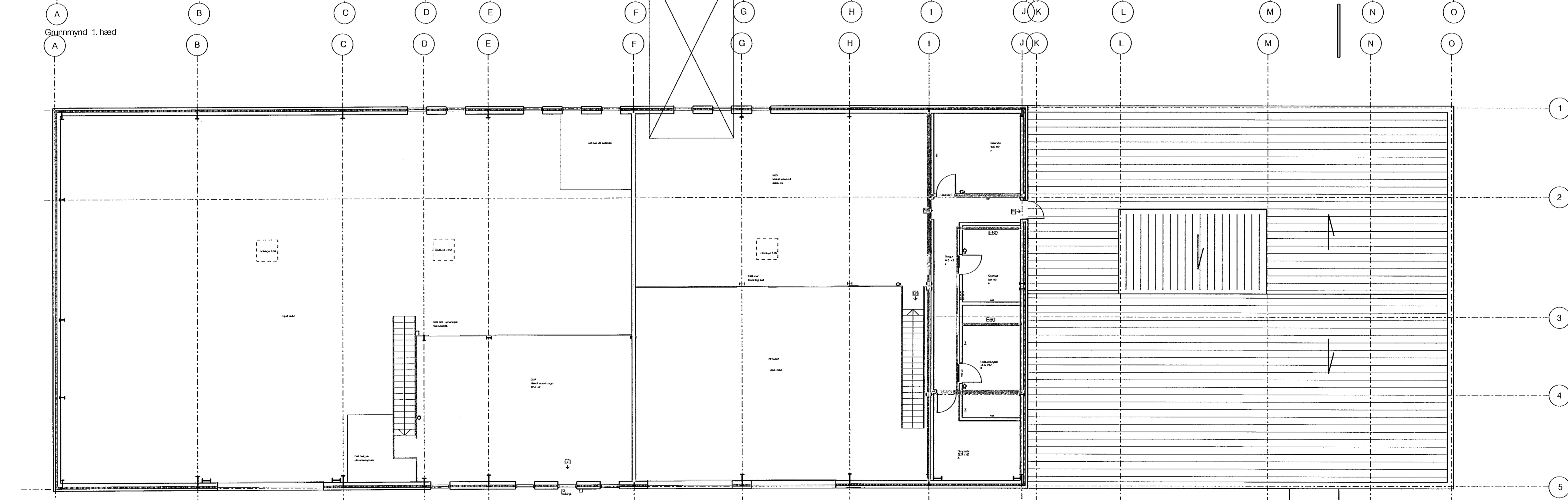
Grunnmynd 2. hæð
