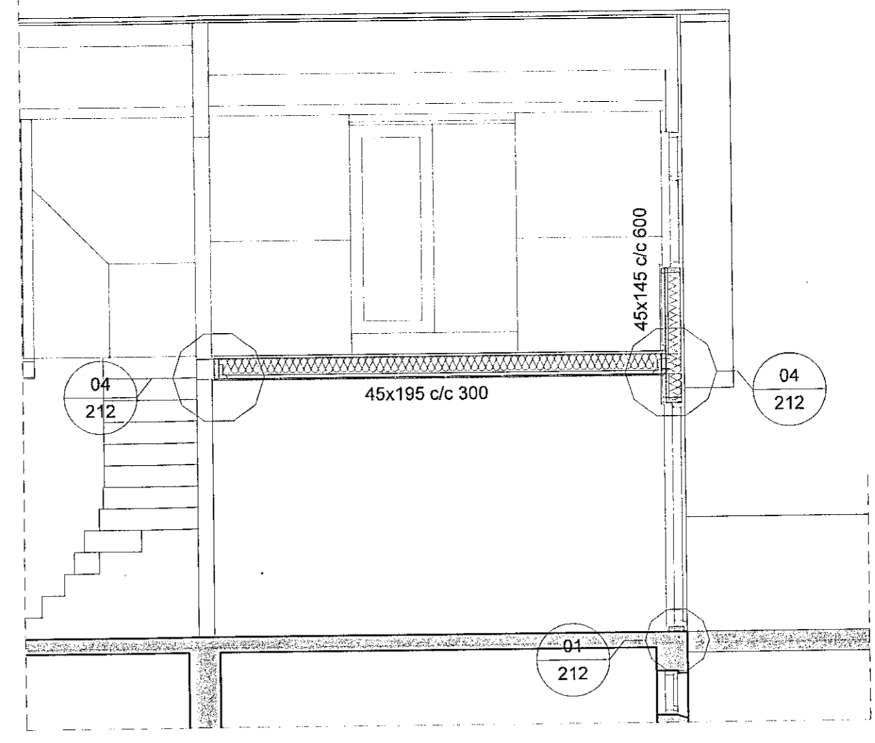
B Snið 211 1:50
