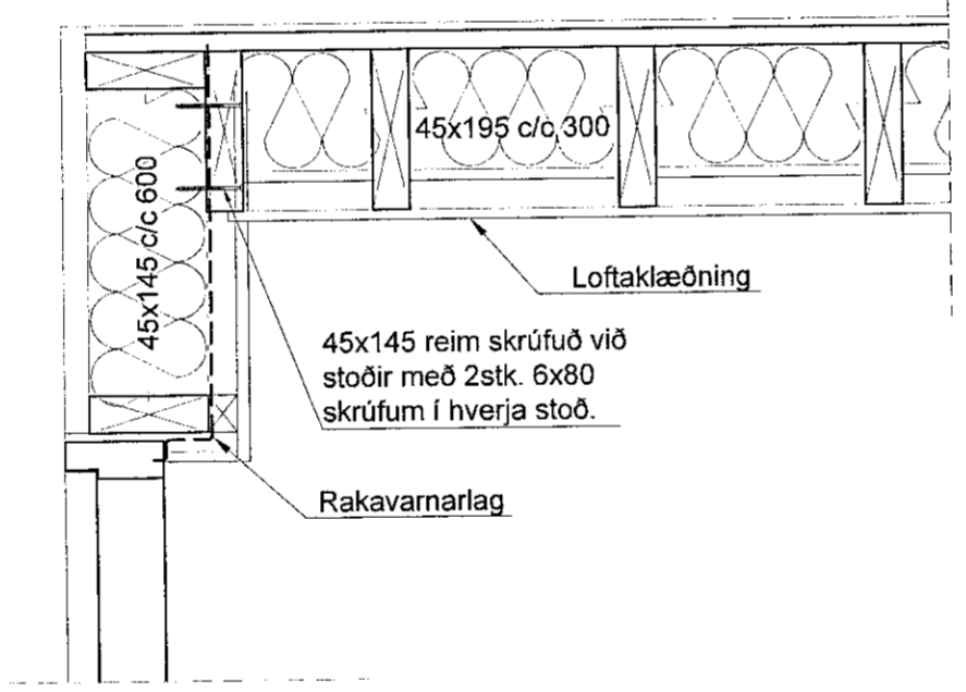
02 Deili 212 1:10
