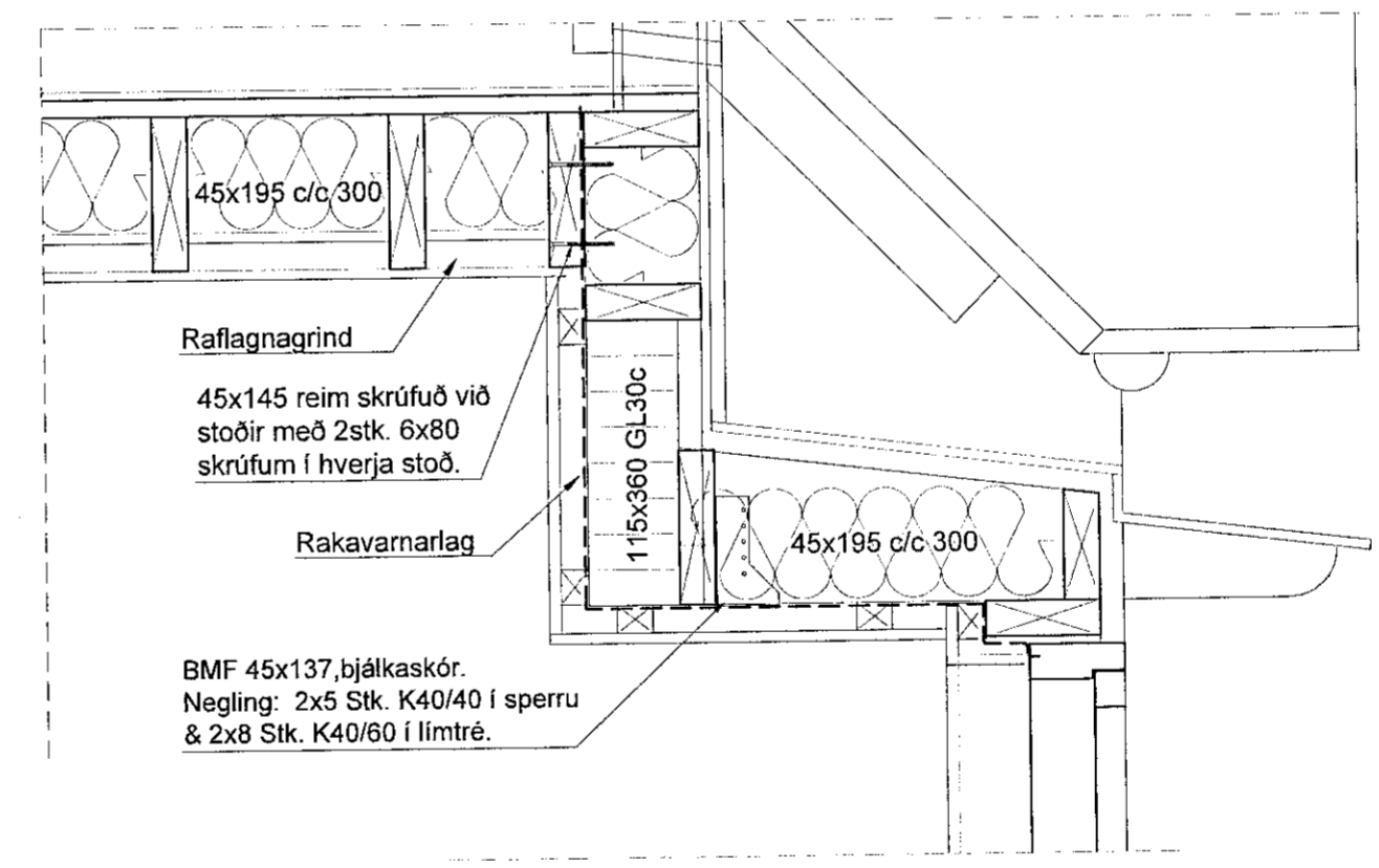
03 Deili 212 1:10
