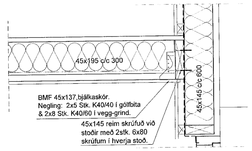
04 Deili 212 1:10
