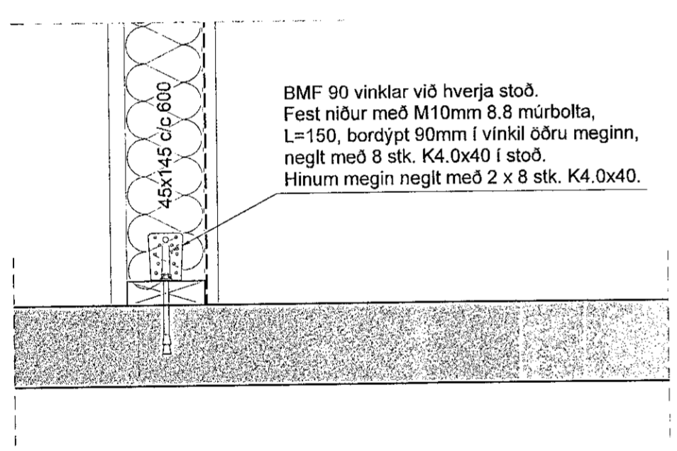
A Snið 211 1:50
