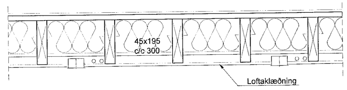
03 Deili 212 1:10
