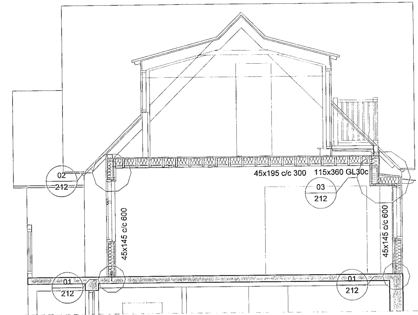
A Snið 211 1:50
