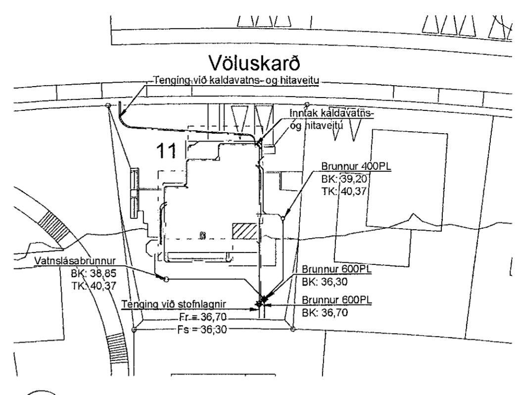
2 Afstöðumynd 1:500
