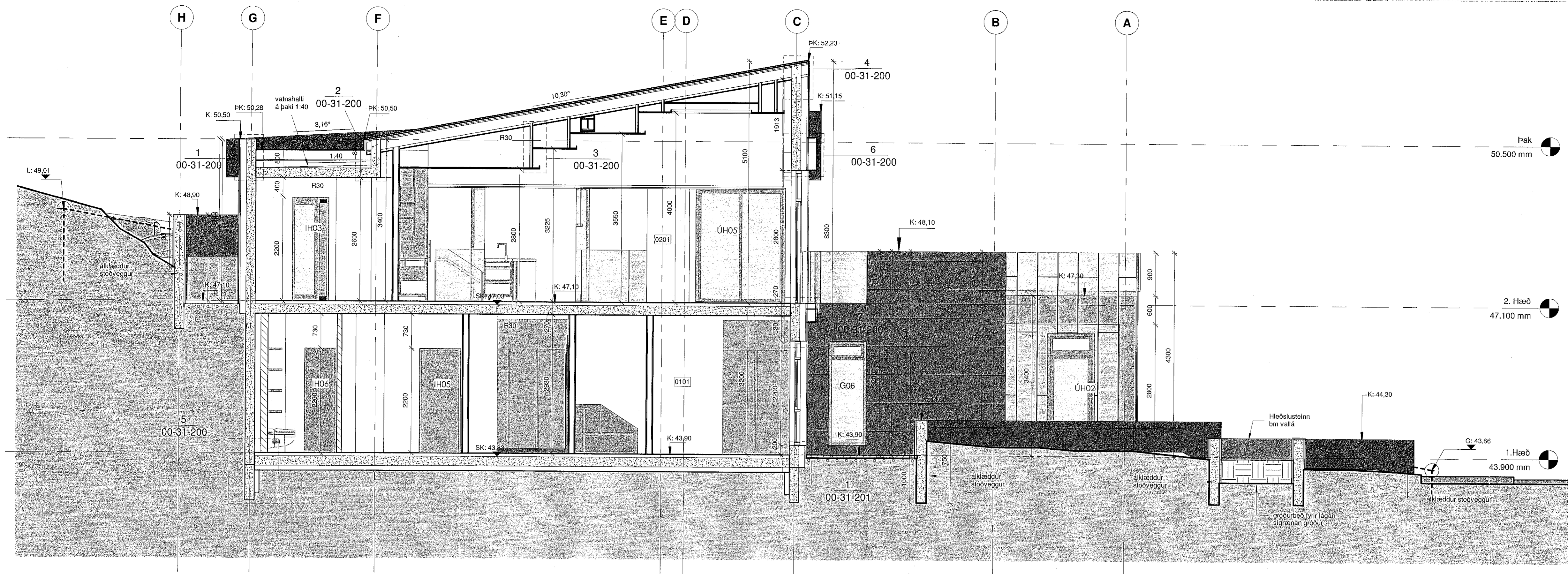
Snið A - 1/50 1 : 50
