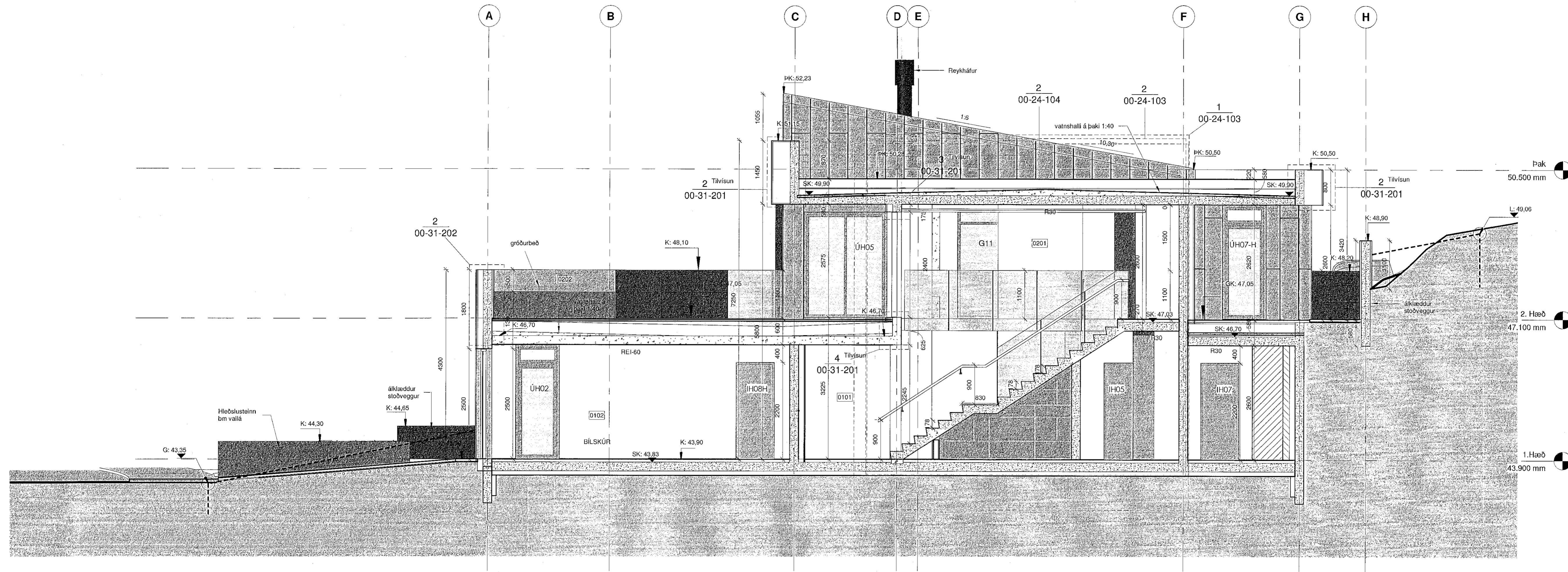
Snið C - 1/50 1 : 50
