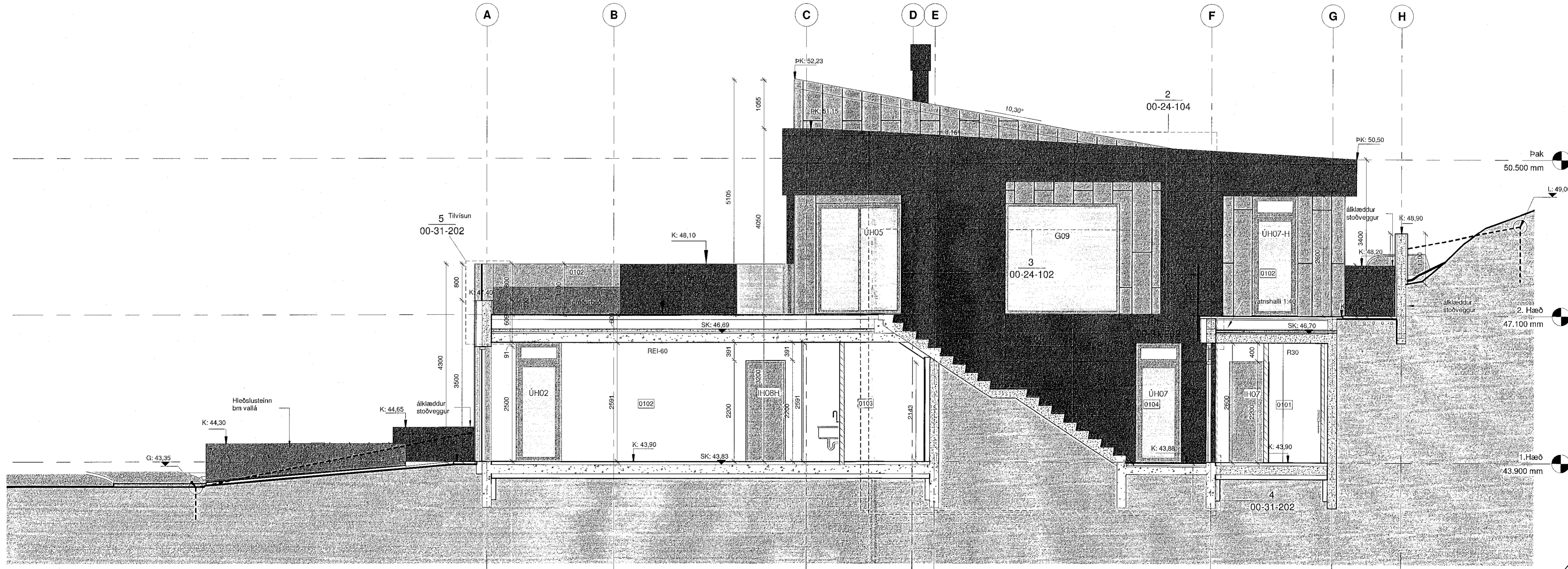
Snið C - 1/50 1 : 50
