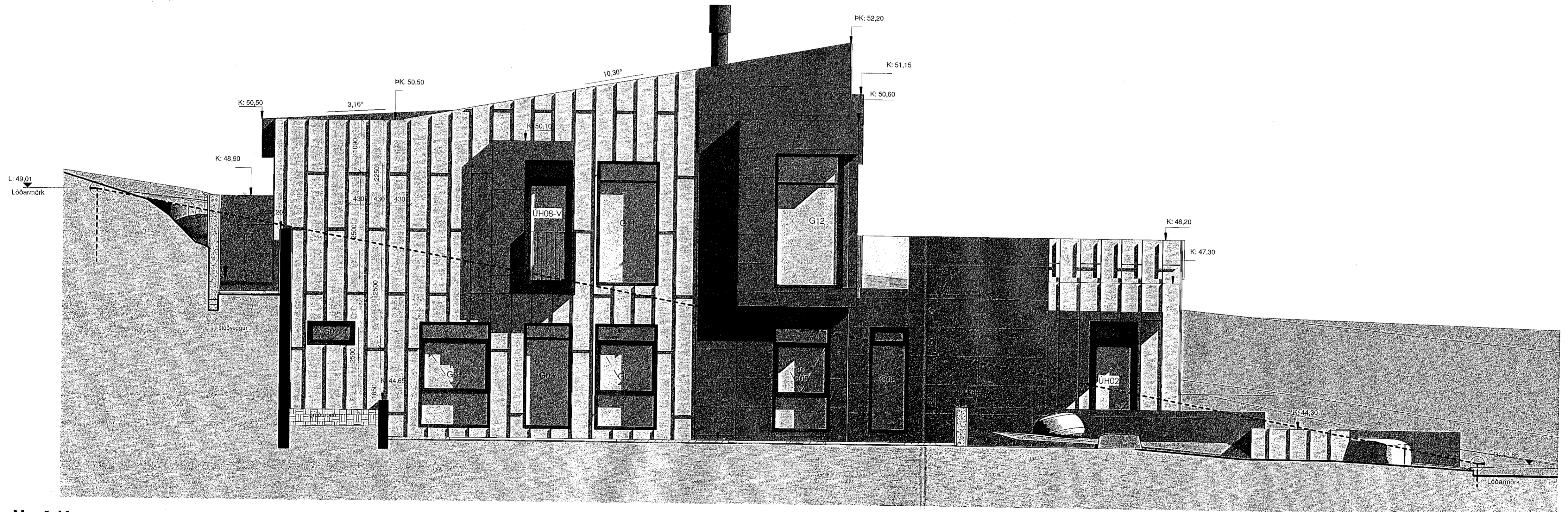
Norð-Vestur 1 : 50
