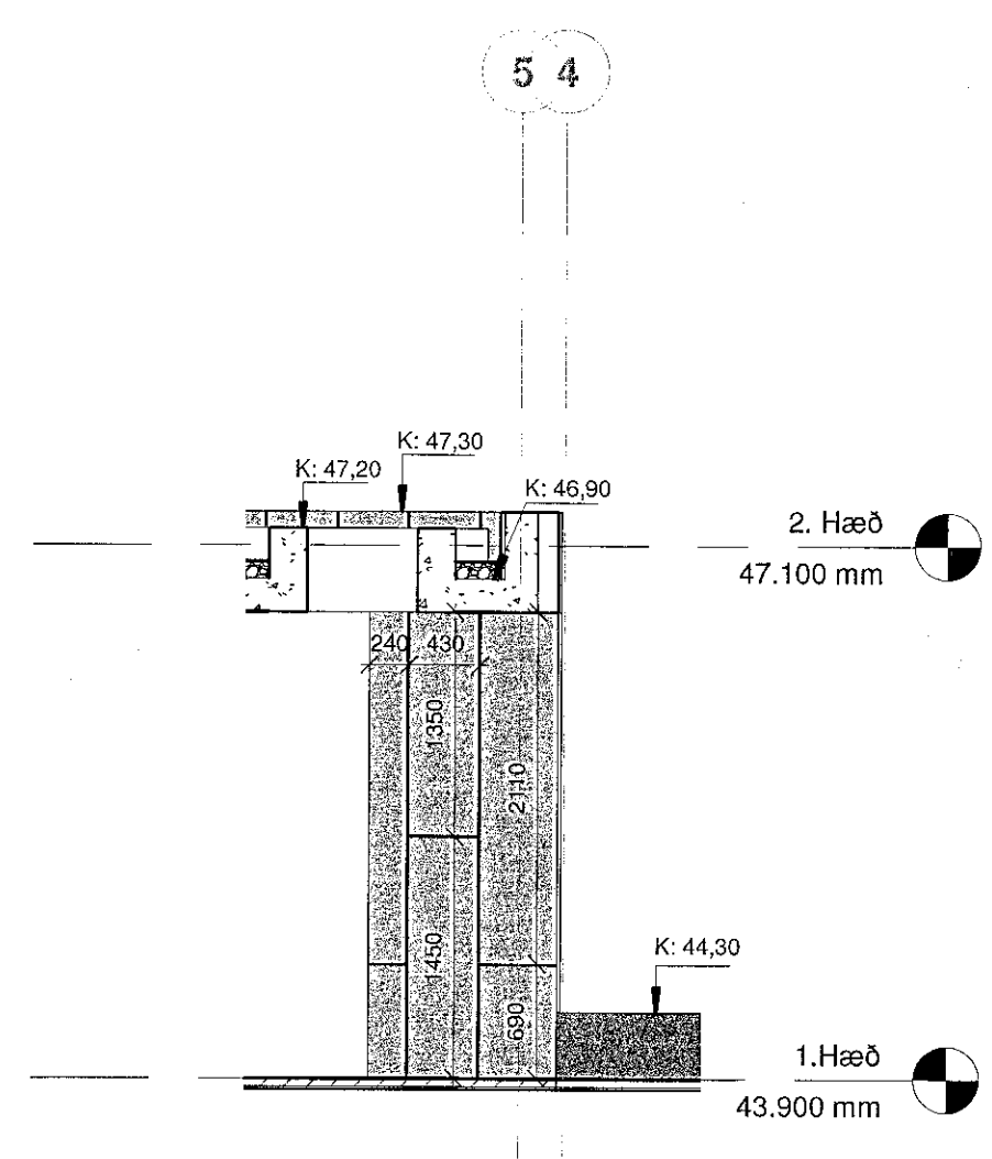
3 Hlutaútlit - Norð-Austur 1/50 súla andyrri 1 : 50
