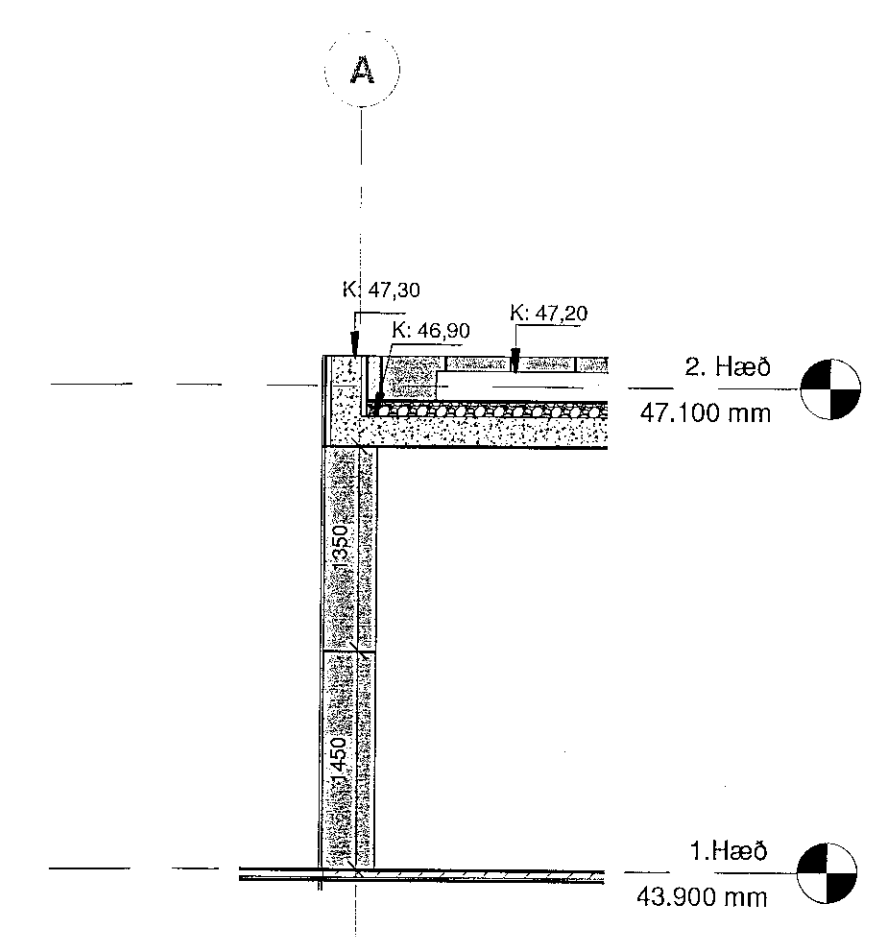
4 Hlutaútlit - Suð-Austur 1/50 súla andyrri 1 : 50
