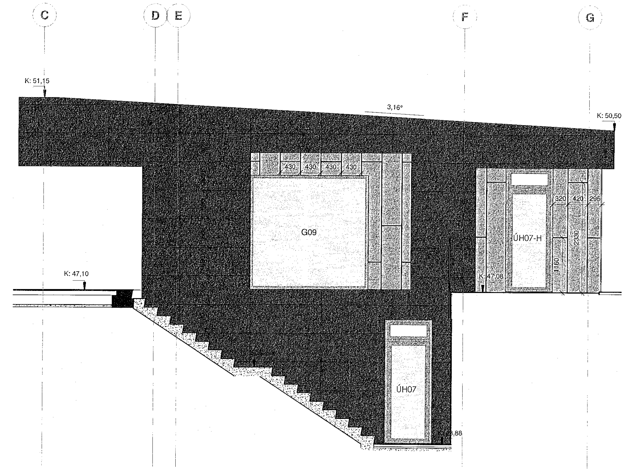
Hlutaútlit - Suð-Austur 1/50 1 : 50
