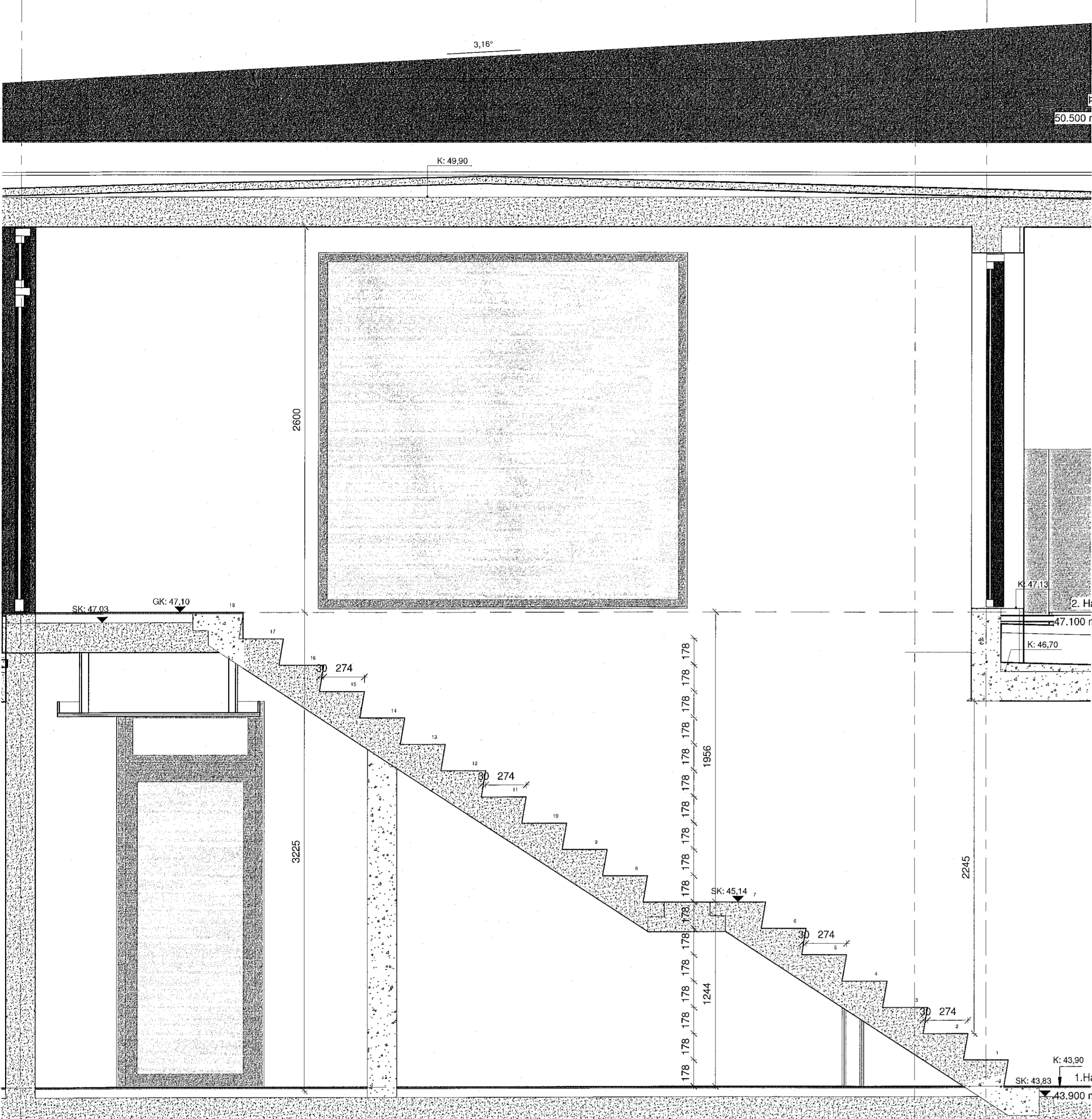
1 Snið A-A Innstigi 1 : 20
