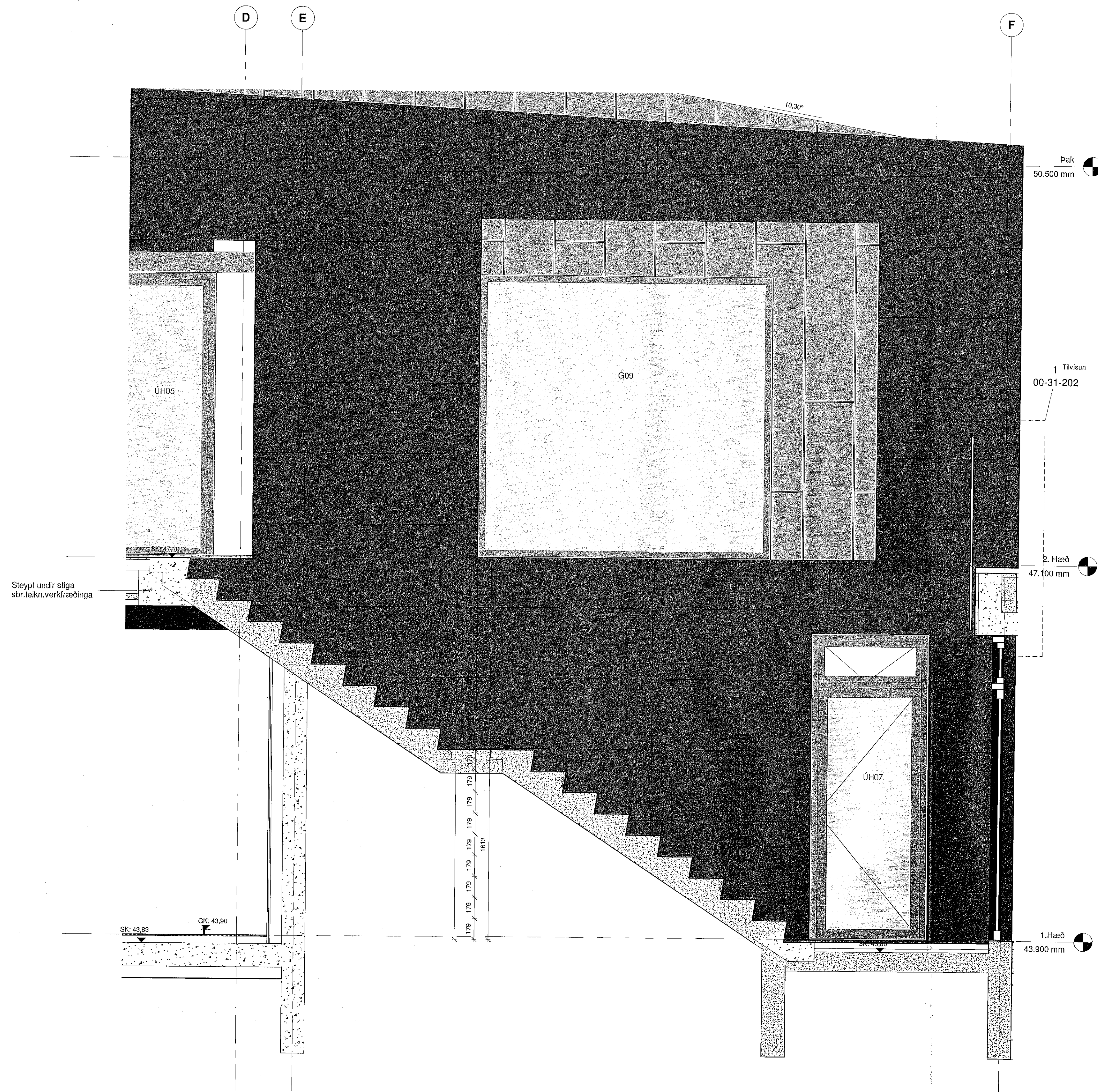
Snið B-B Útistigi 1 : 20
