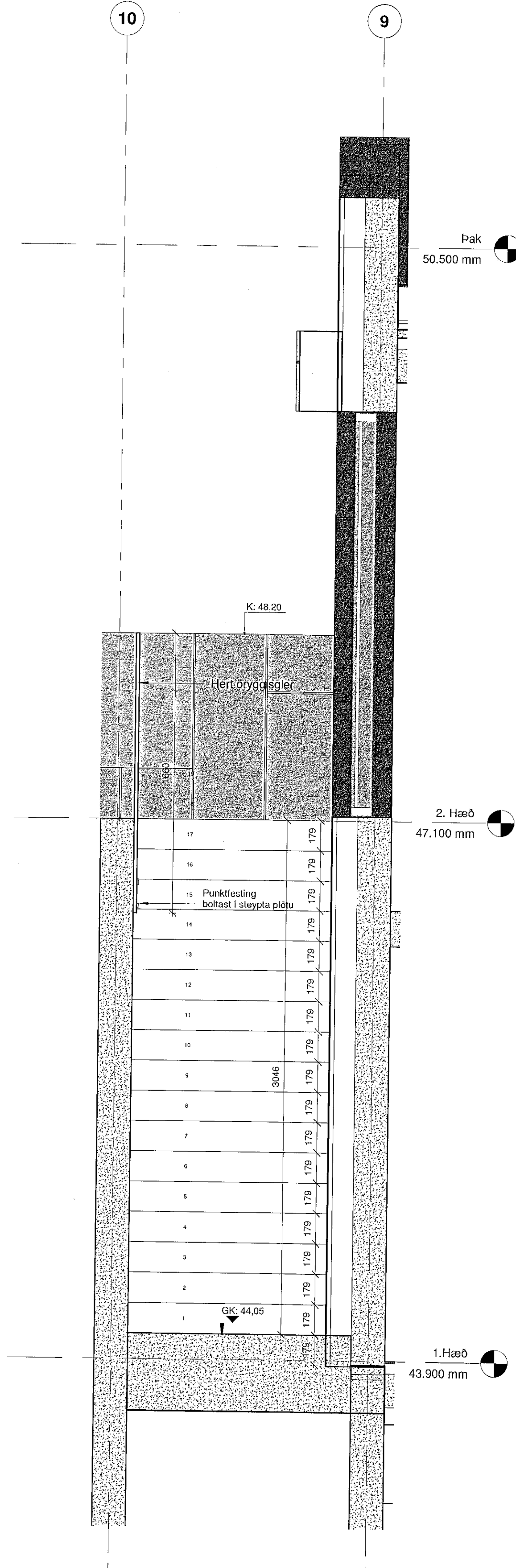
1 Snið C-C Útistigi 1 : 20
