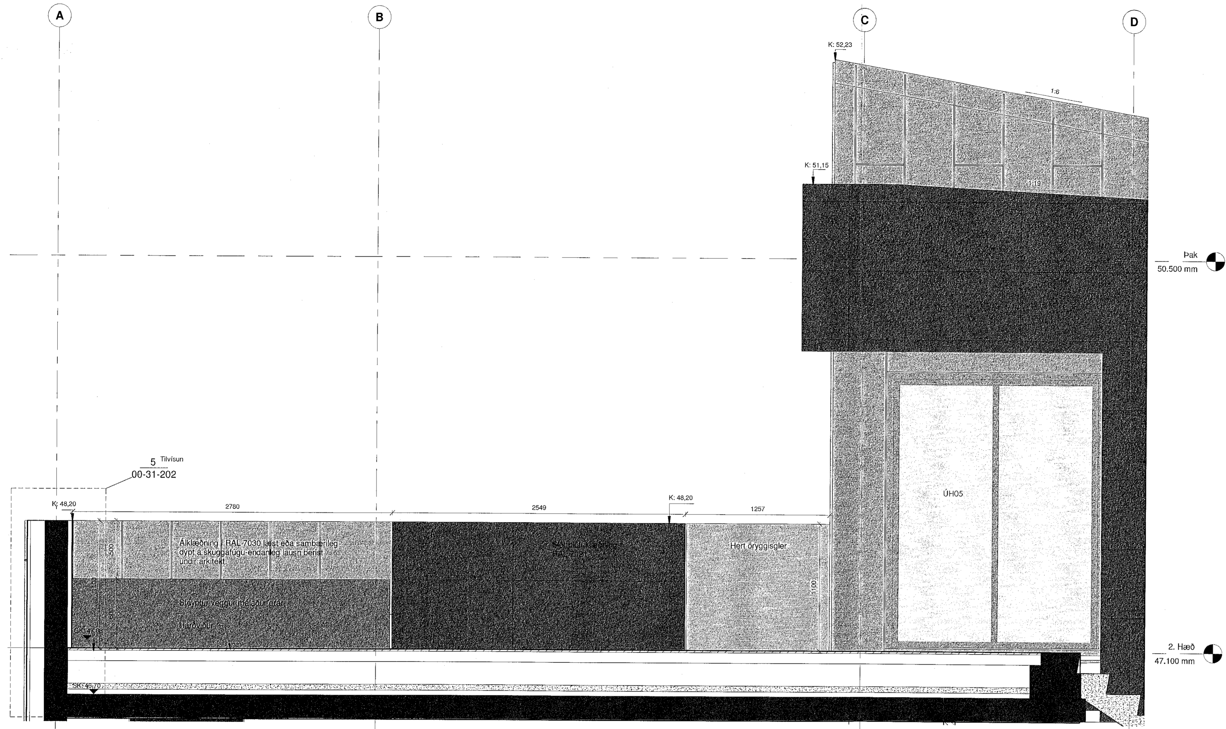
Svalir - Hluti 1 - Snið A-A 1 : 20
