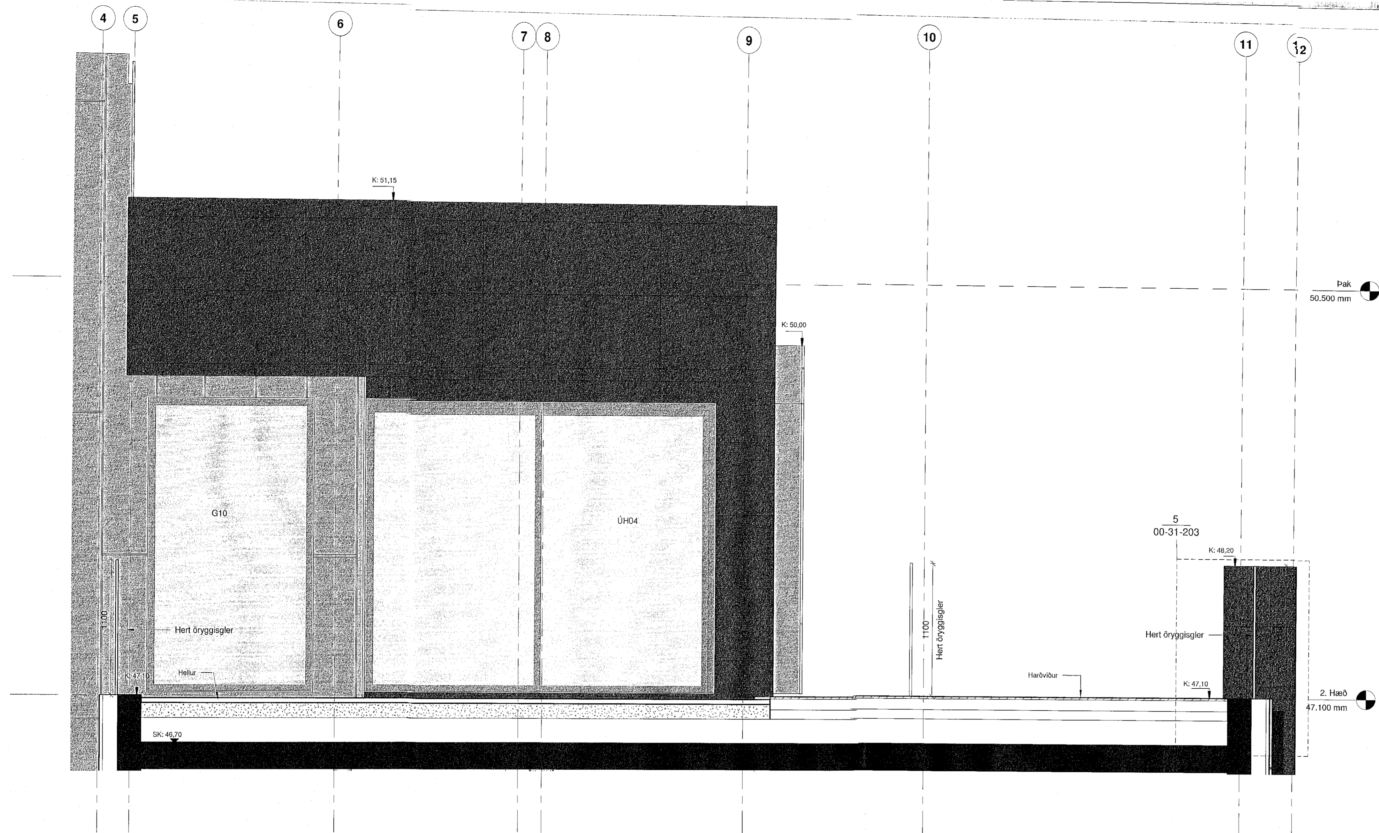
Svalir - Hluti 1 - Snið C-C 1 : 20
