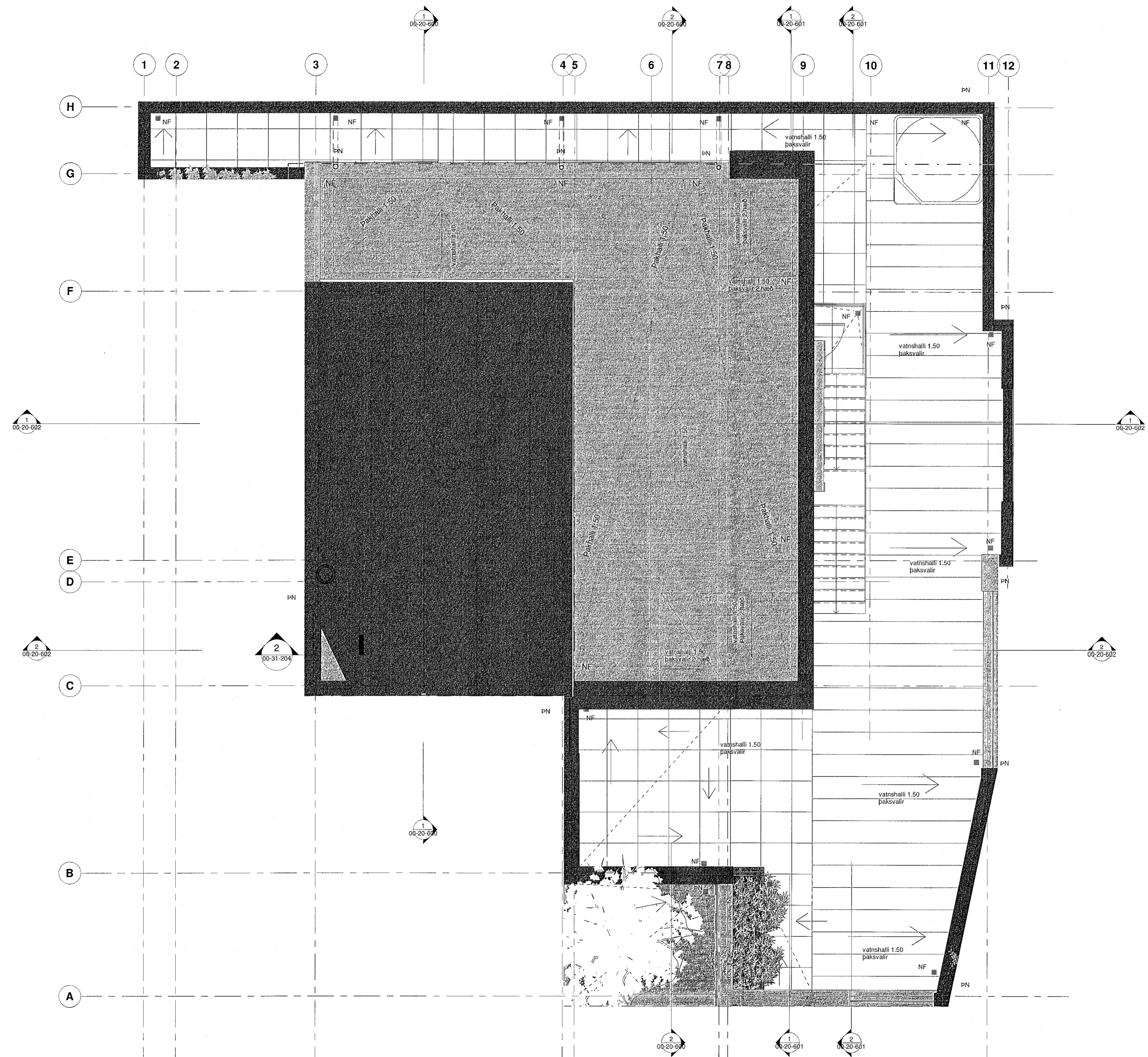
Grunnmynd þakhallaplan 1 : 50
