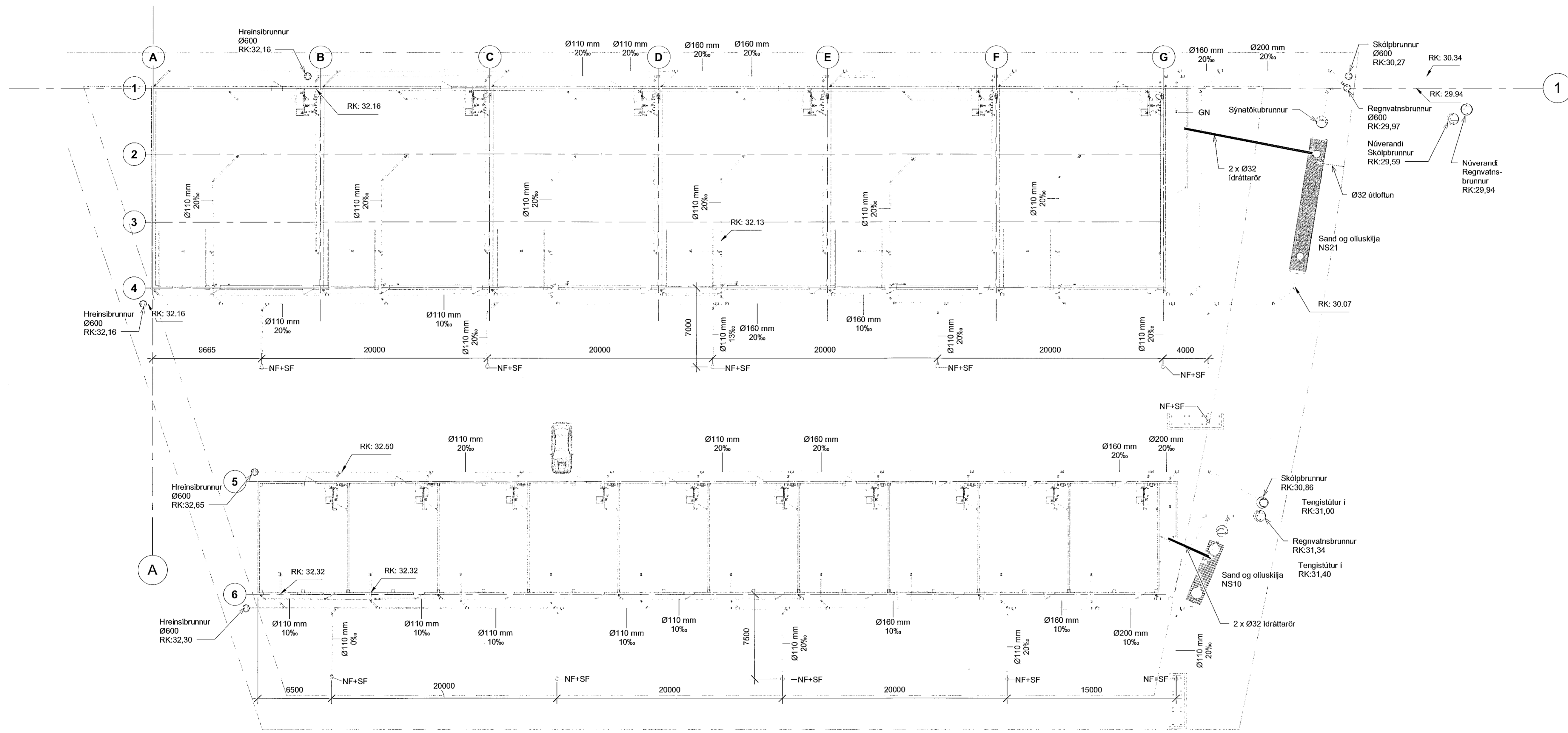
1 Yfirlitsmynd lagna á lóð 1 : 200
