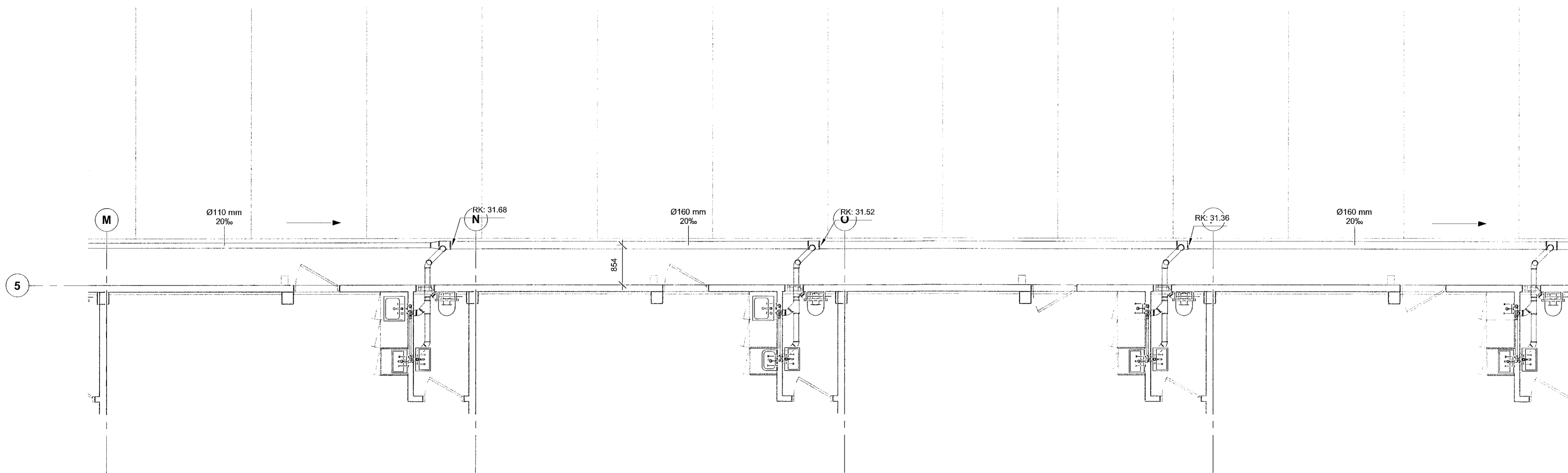
1 Grunnmynd, lagnir á lóð 1:50
