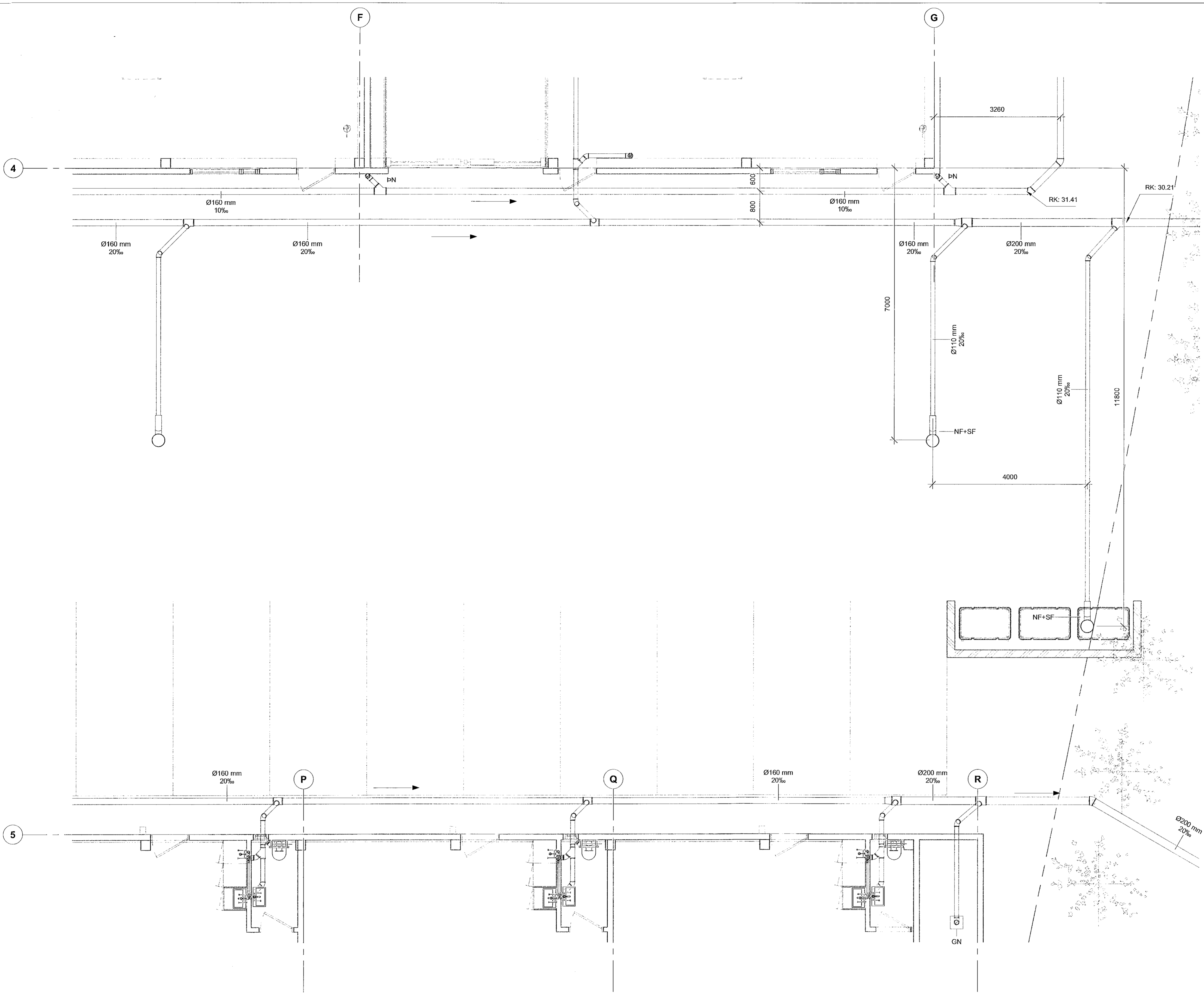
1 Grunnmynd, lagnir á lóð 1 : 50
