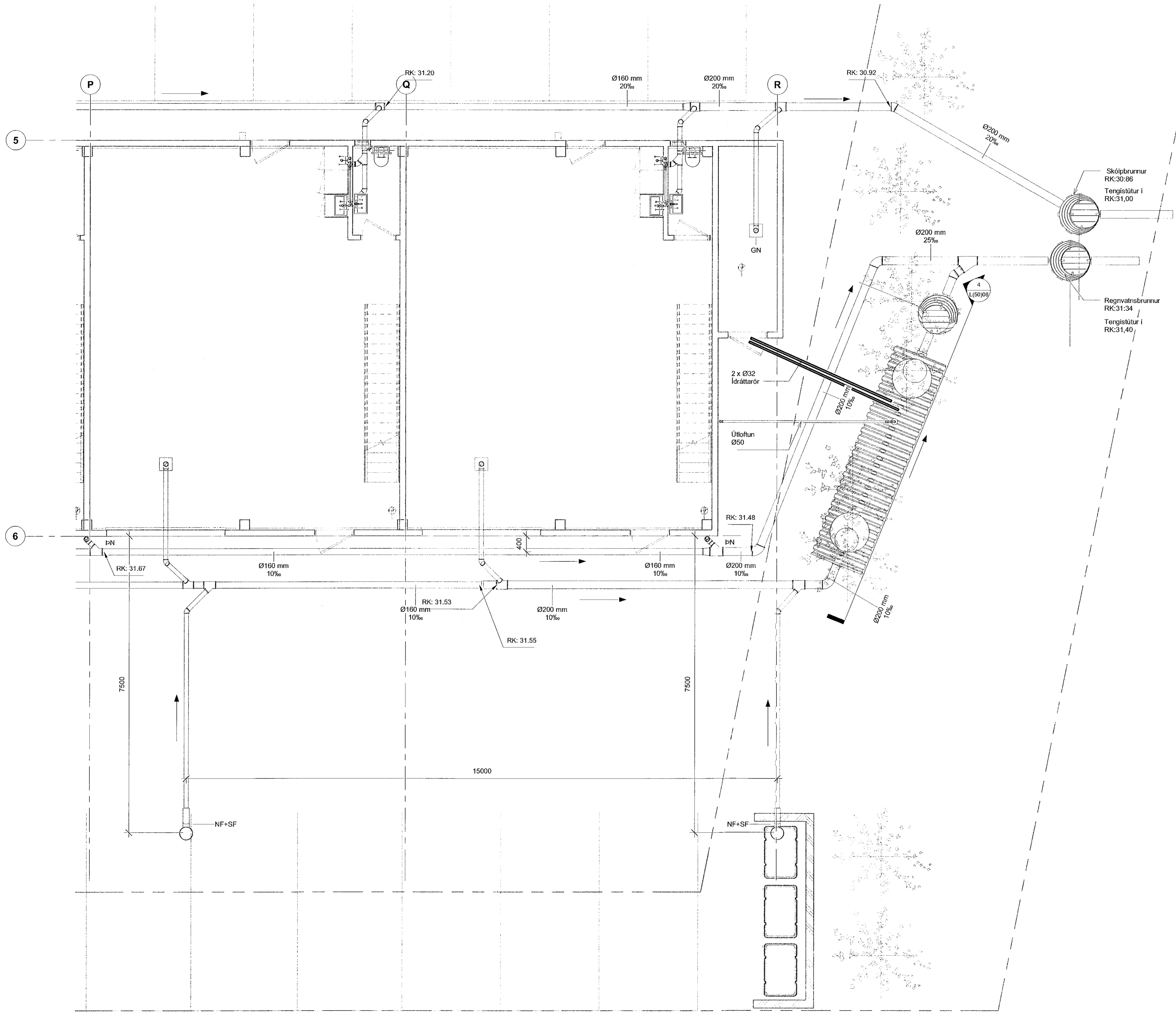
1 Grunnmynd, lagnir á lóð 1:50
