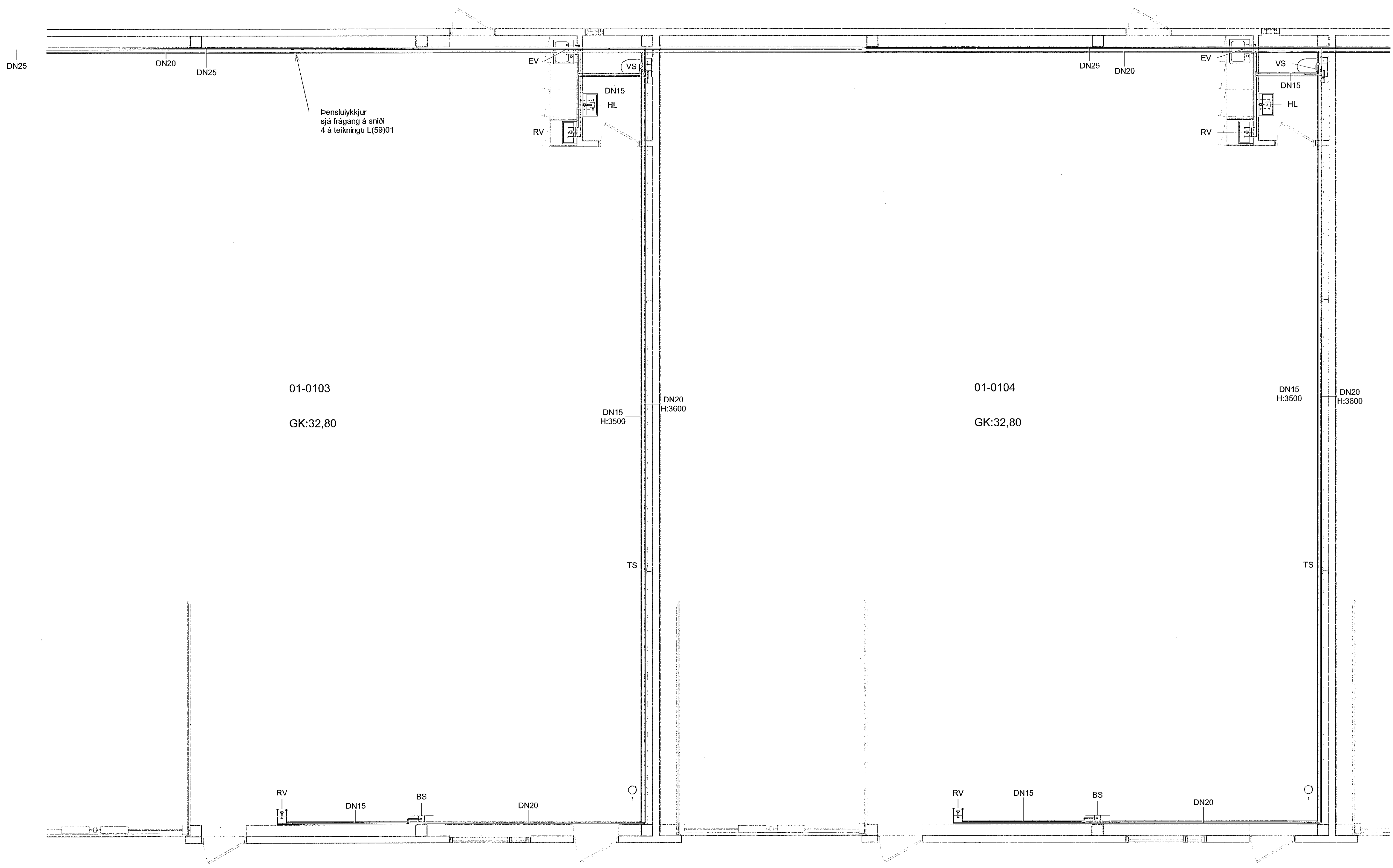
1 Grunnmynd 1. Hæð 1:50
