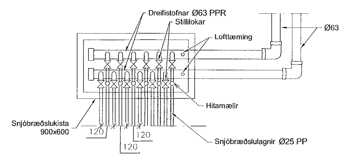
2 Snjóbræðslukista 1 : 20
