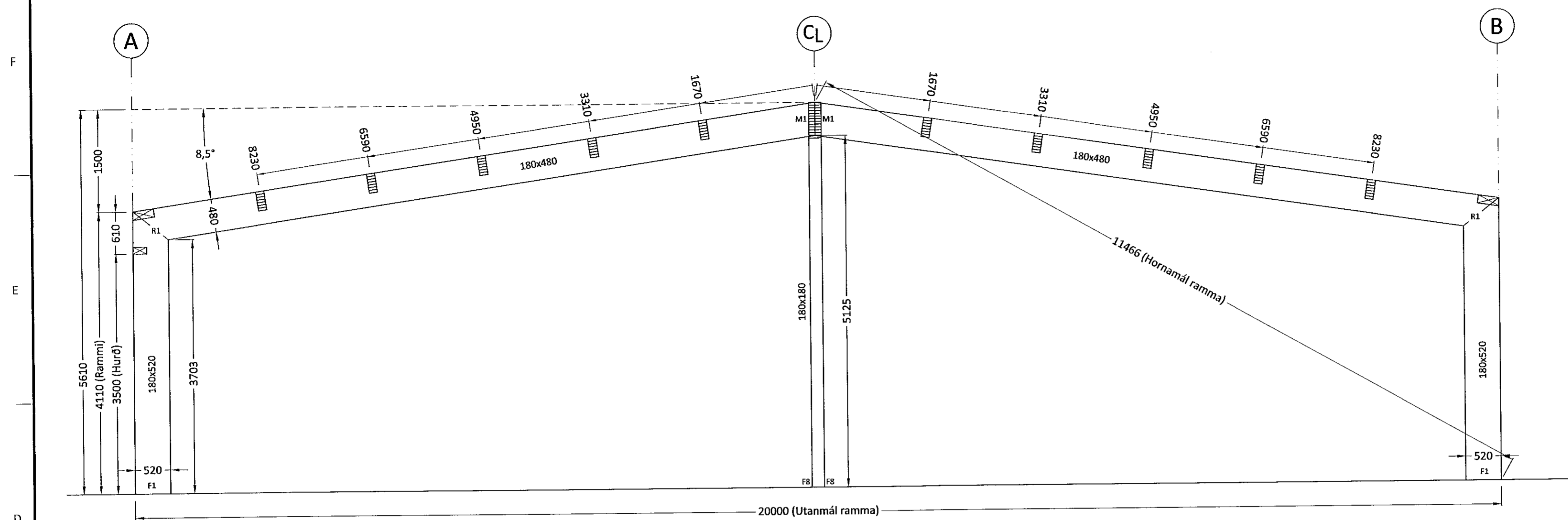
MODULE - 2-6 Mkv. 1:50
