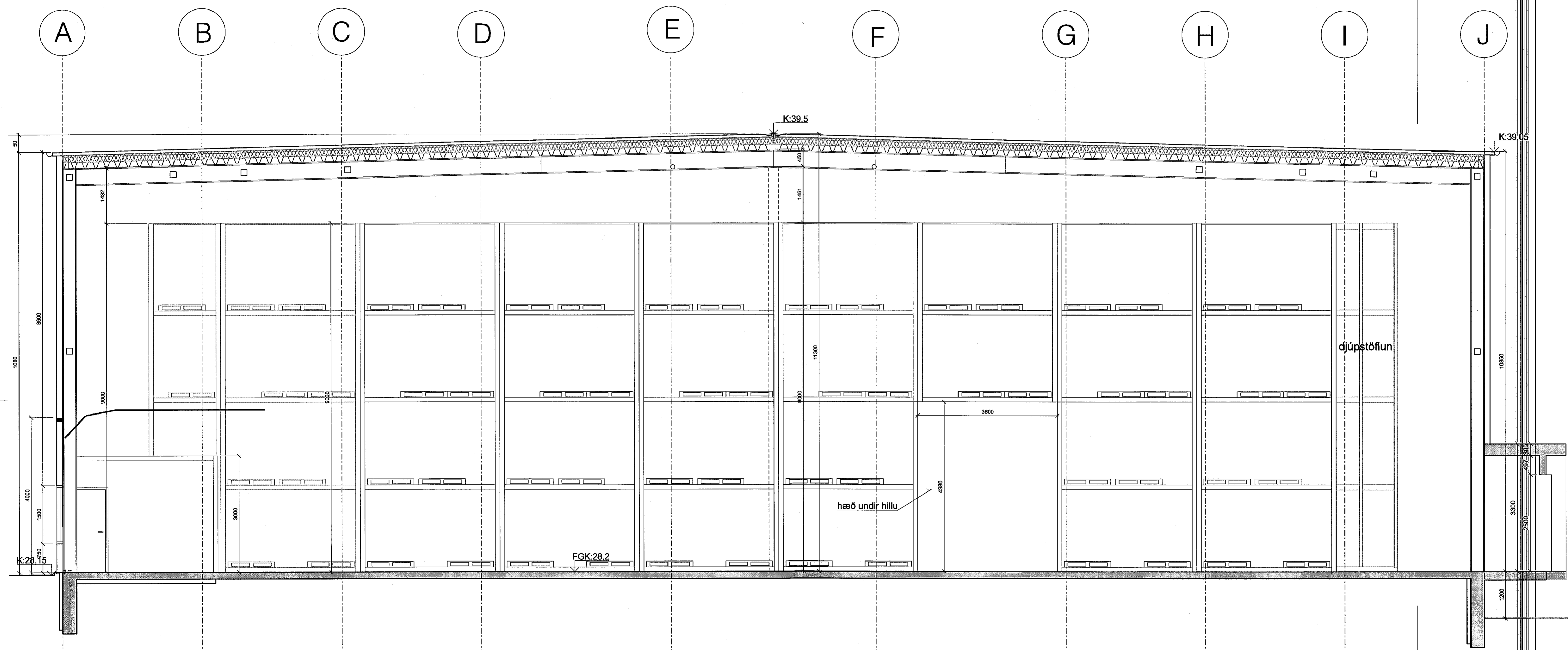
A-A 20-05 SNEIÐING 1:50
