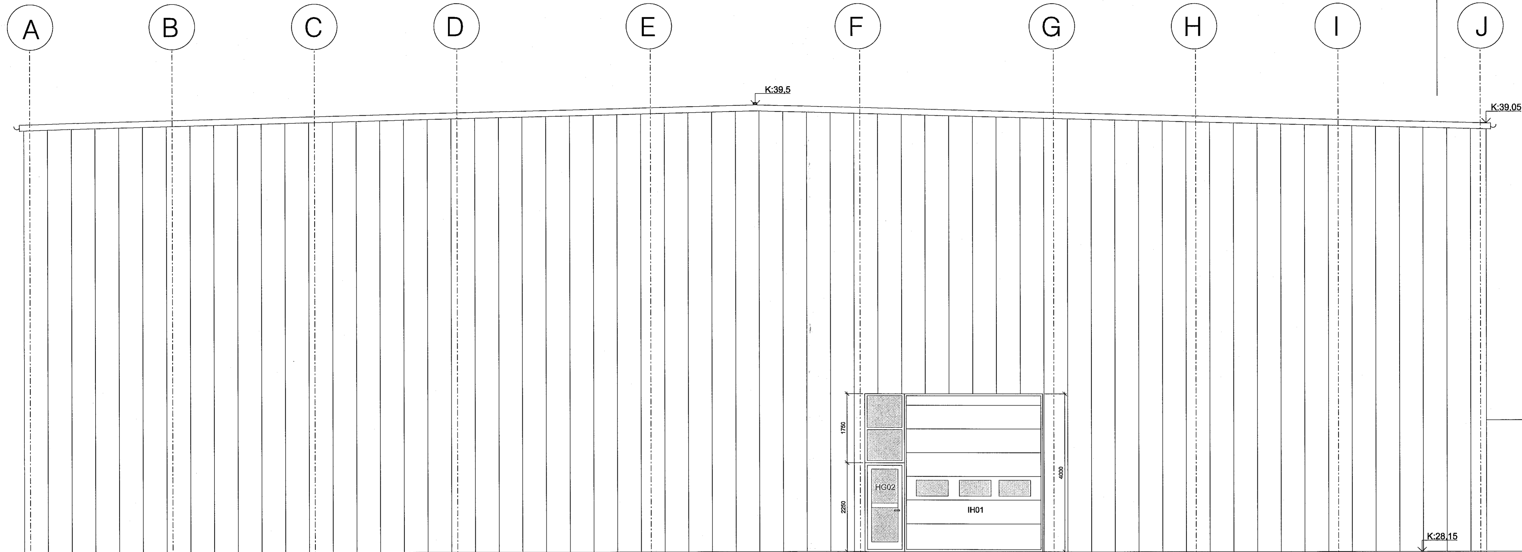
ÚTLIT 1:50 AUSTUR
