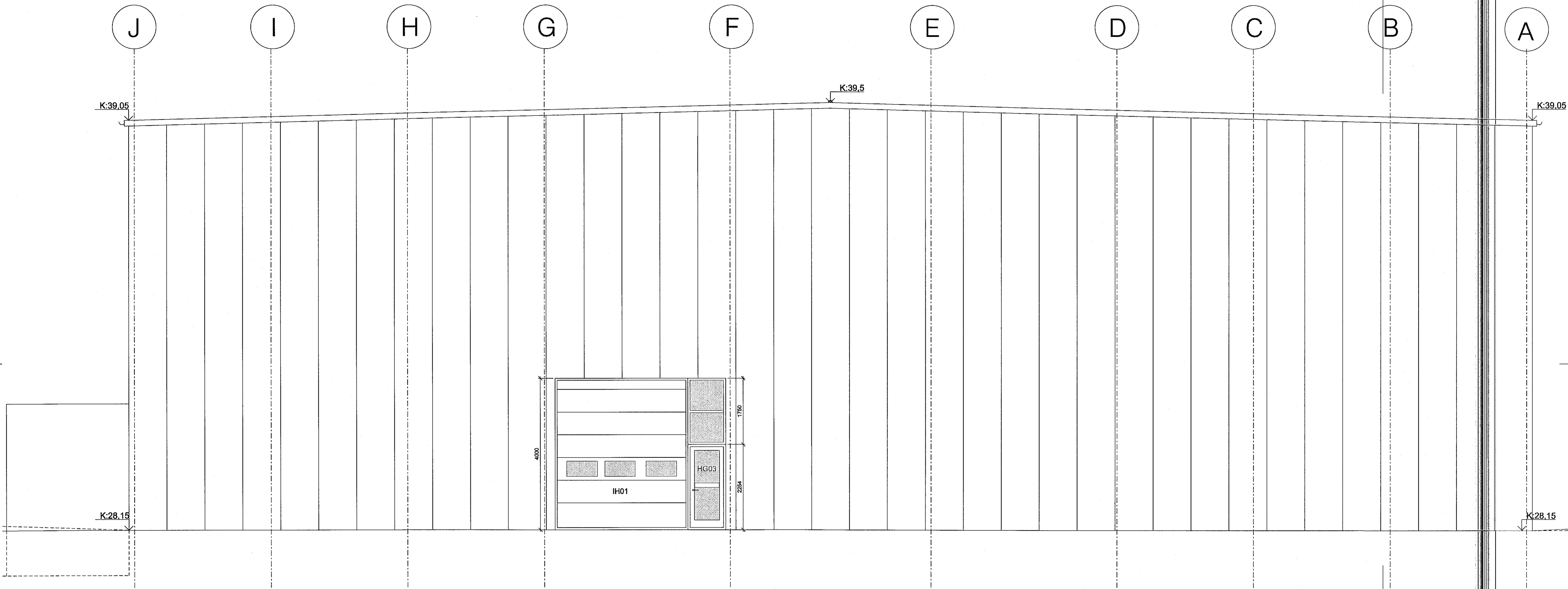
ÚTLIT 1:50 VESTUR
