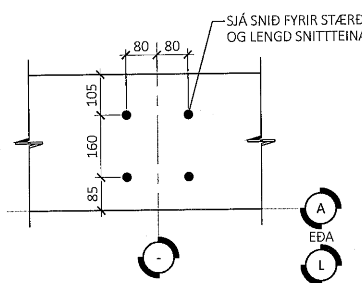
INNSTEYPTIR SNITTEINAR Á LANGHLÍÐUM - M1:10:
