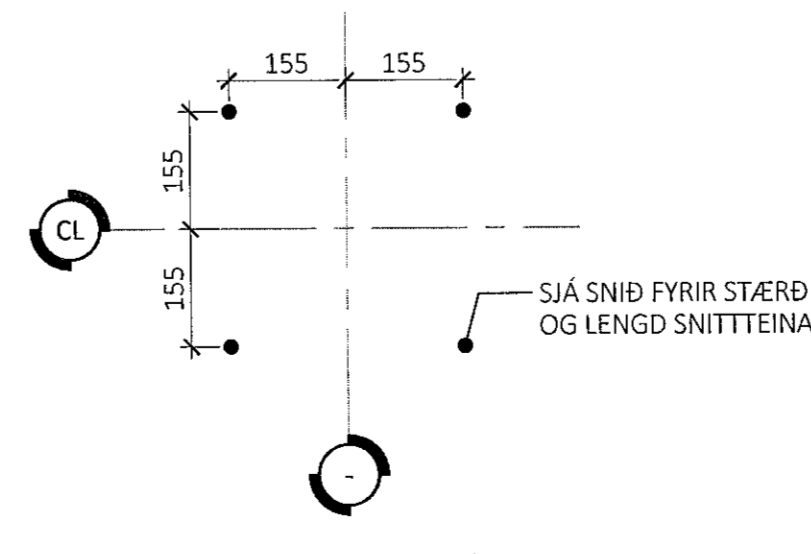
INNSTEYPTIR SNITTEINAR FYRIR SÓLUR Í MÁTLÍNU CL - M1:5:
