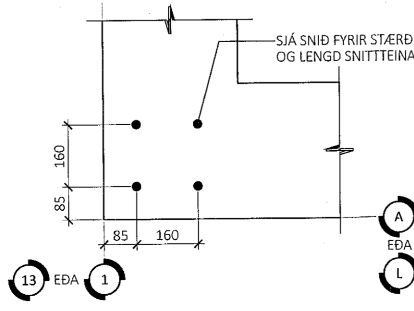
INNSTEYPTIR SNITTEINAR Á HORNUM - M1:5:
