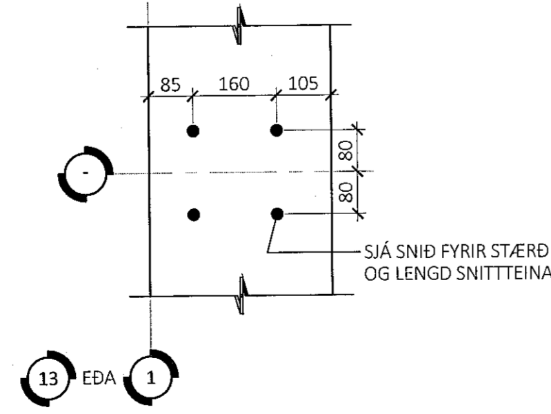
INNSTEYPTIR SNITTEINAR Á SKAMMHLÍÐUM - M1:5:
