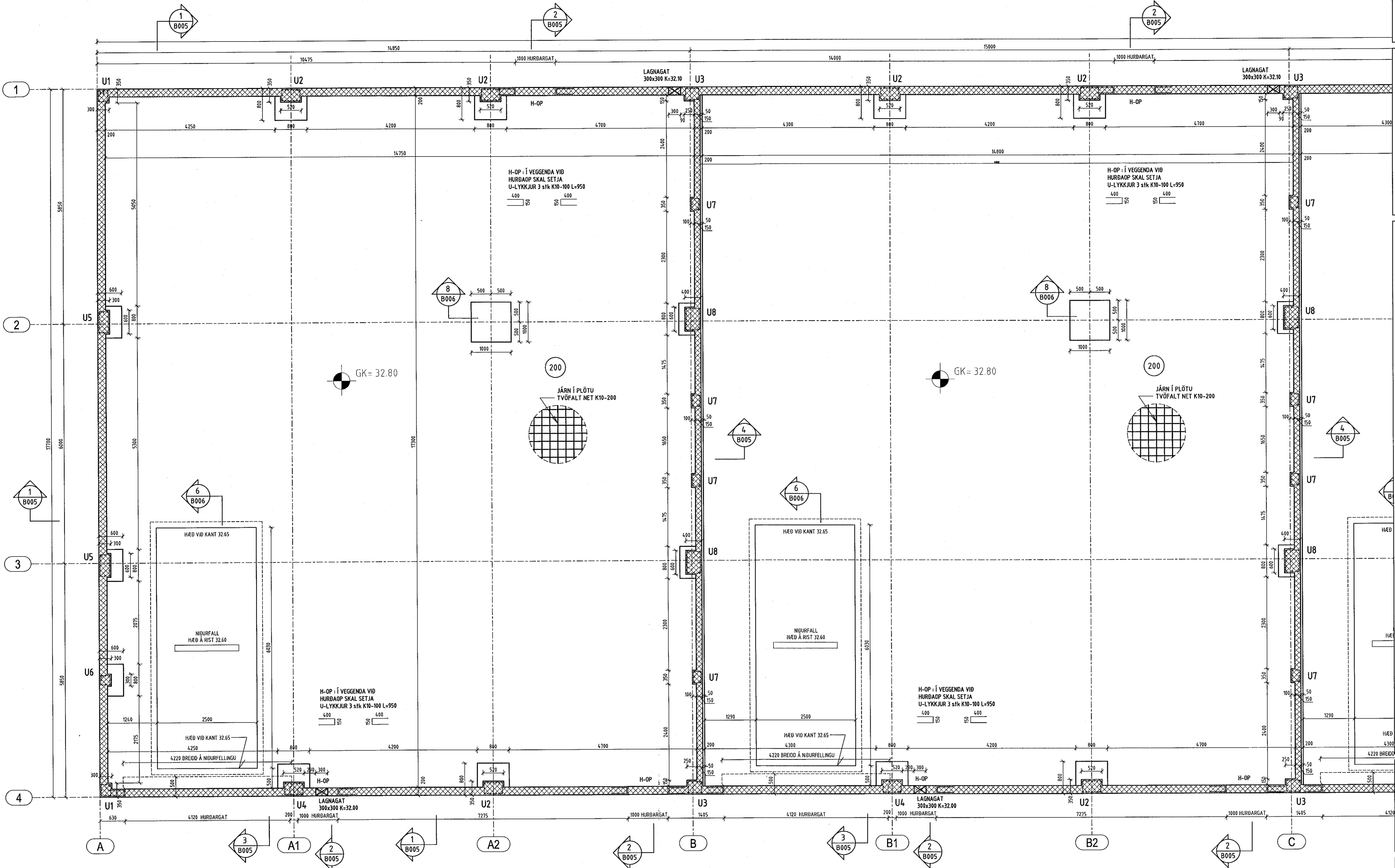
UNDIRSTÖÐUR GRUNNMYND 1:50
