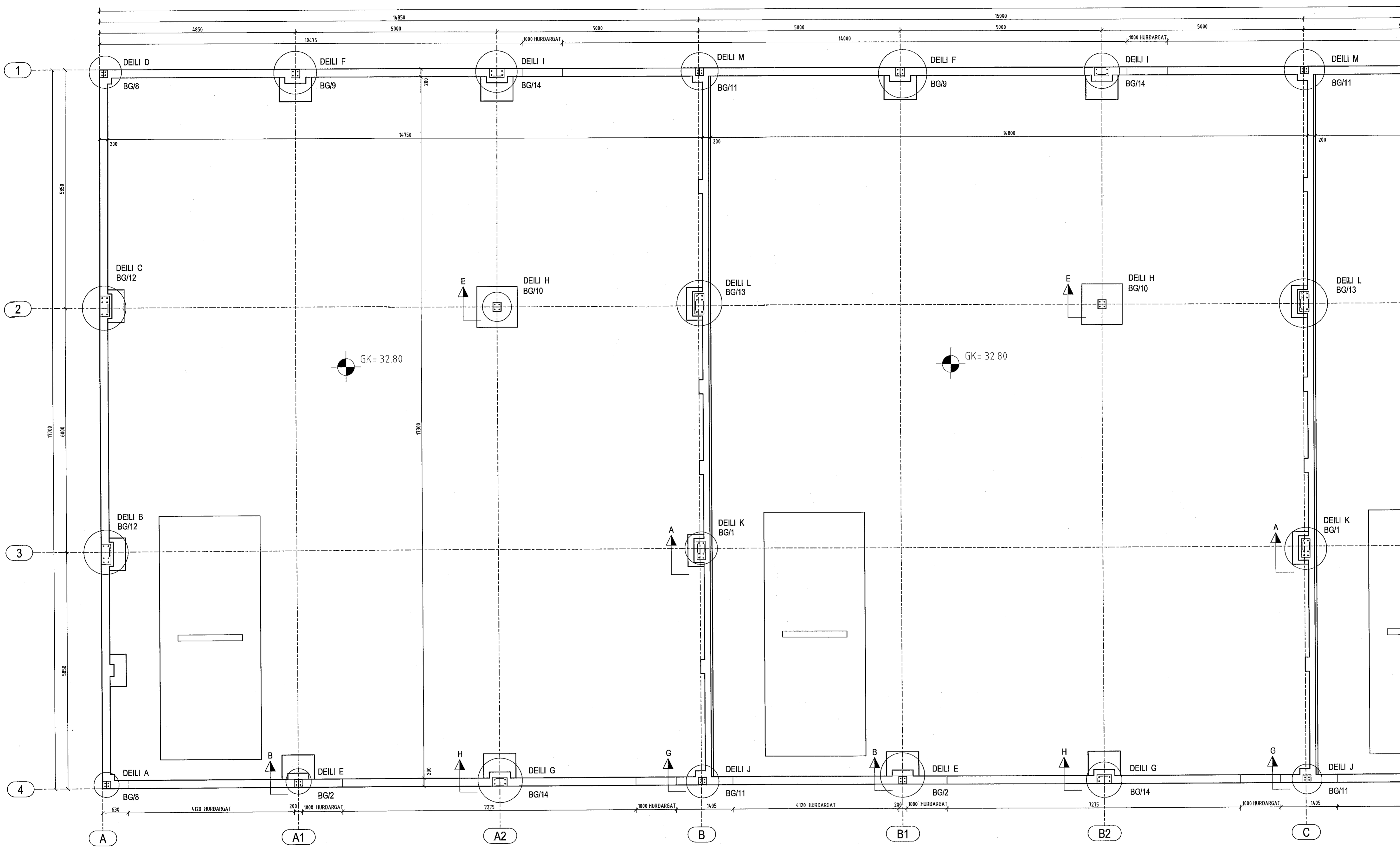
INNSTEYPTIR BOLTAR BURÐARSÚLUR 1:50
