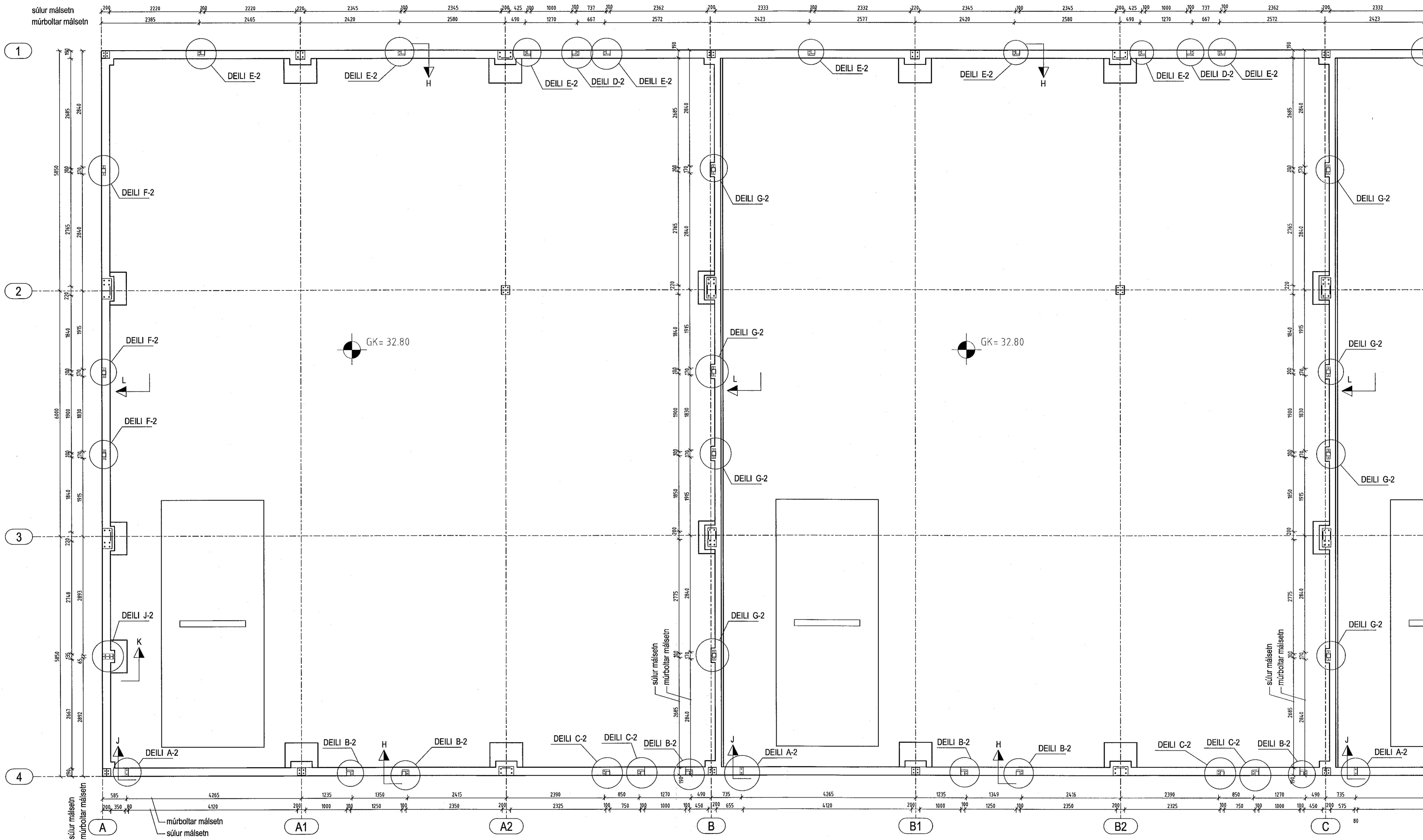
MÚRBOLTAR MILLISÚLUR 1:50
