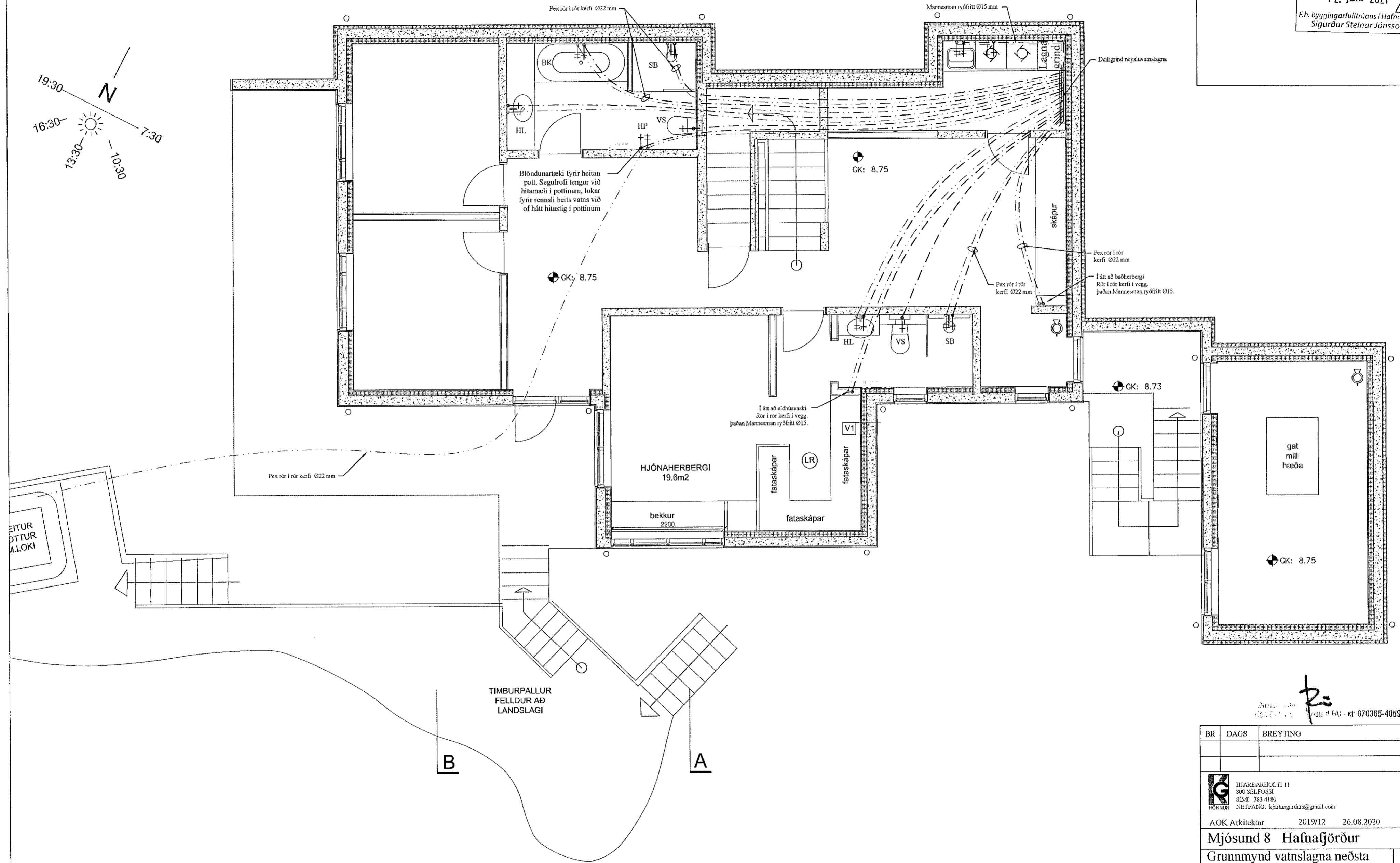
Grunnmynd neysluvatnslagna neðsta hæð MKV: 1:50
