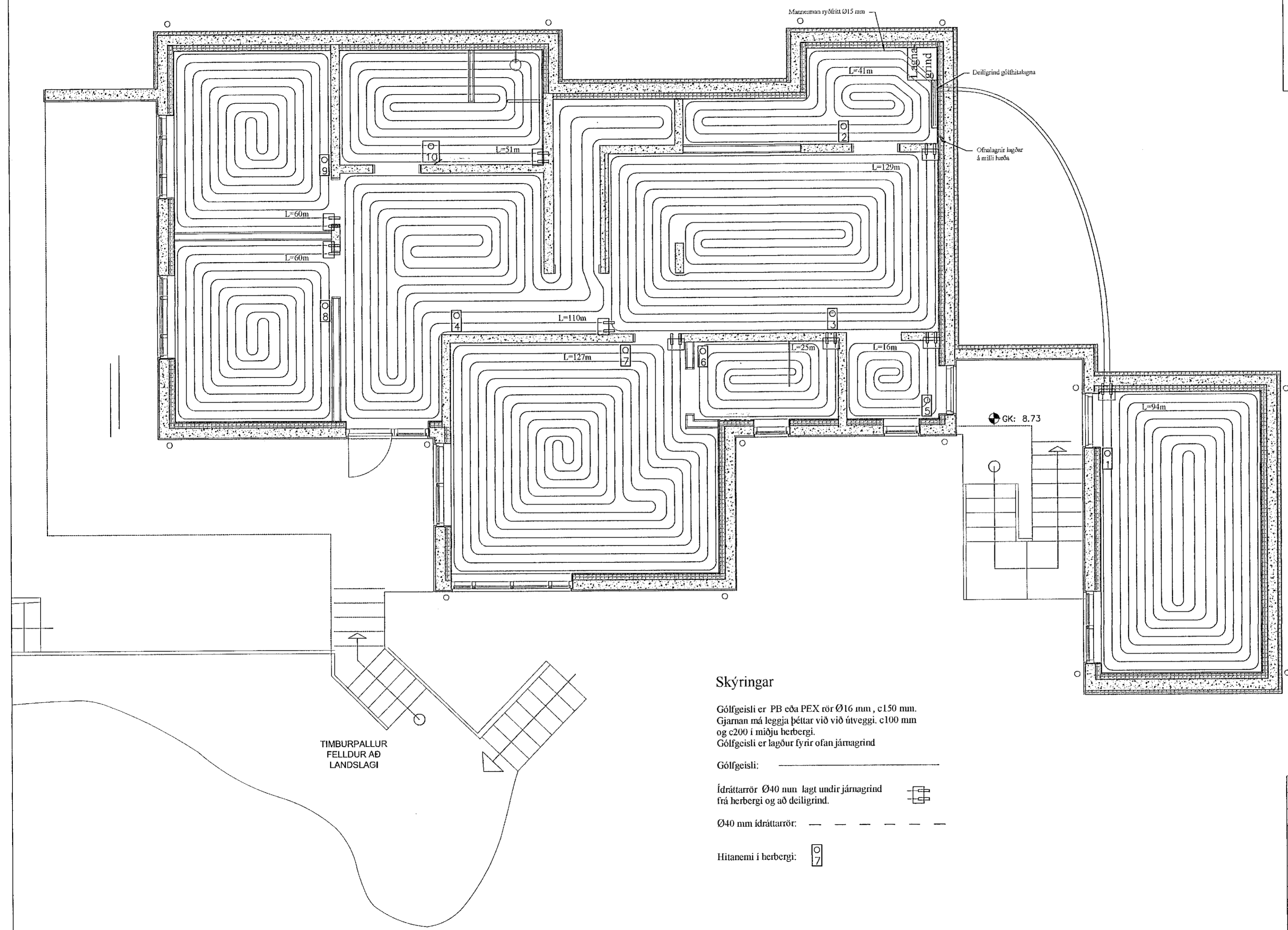
Grunnmynd hitalagna neðsta hæð MKV: 1:50
